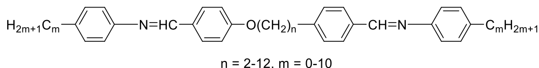
Slika 14. Struktura \alpha,\omega -bis[4-(4'-alkilfeniliminometil)fenil]oksialkana.
