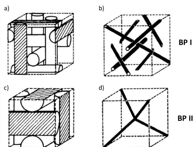
Slika 23. Prikaz struktura plavih faza I i II. Lokalno slaganje dvostrukih cilindara prikazano je pod a) i c) dok je pod b) i d) dan prikaz disklinacijskih linija. 99
