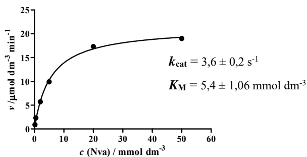
Slika 4.15: Michaelis-Mentetin prikaz ovisnosti početne brzine o koncentraciji supstrata (norvalina) u reakciji kataliziranoj enzimom hsLeuRS. Prikazana je srednja vrijednost tri neovisna mjerenja. Reakcije su mjerene u uvjetima ustaljenog stanja.
