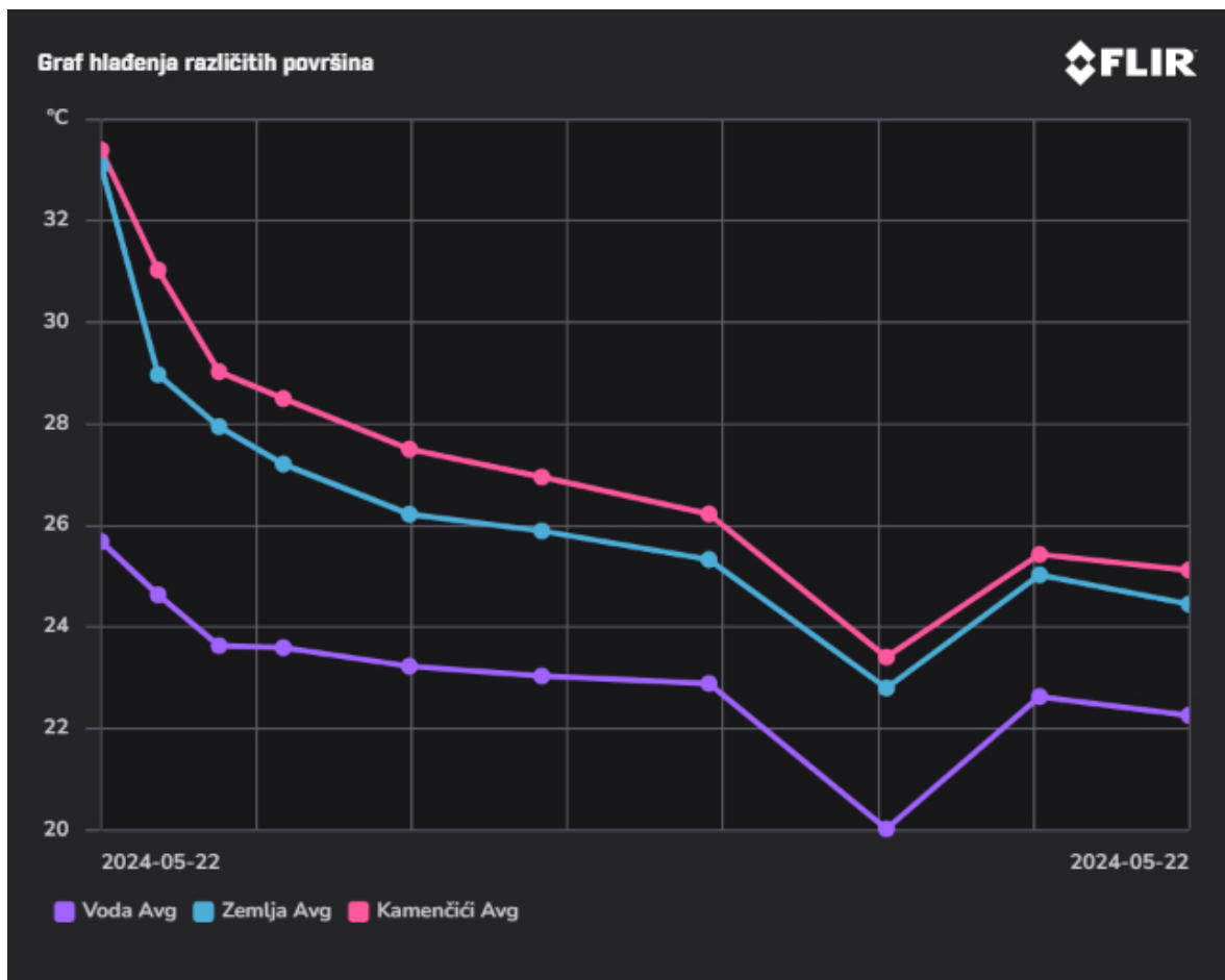
Slika 4.9: Graf hlađenja različitih površina
