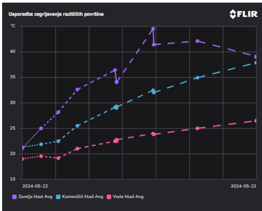
Slika 4.4: Usporedba zagrijavanja površina - slikano u hladu
