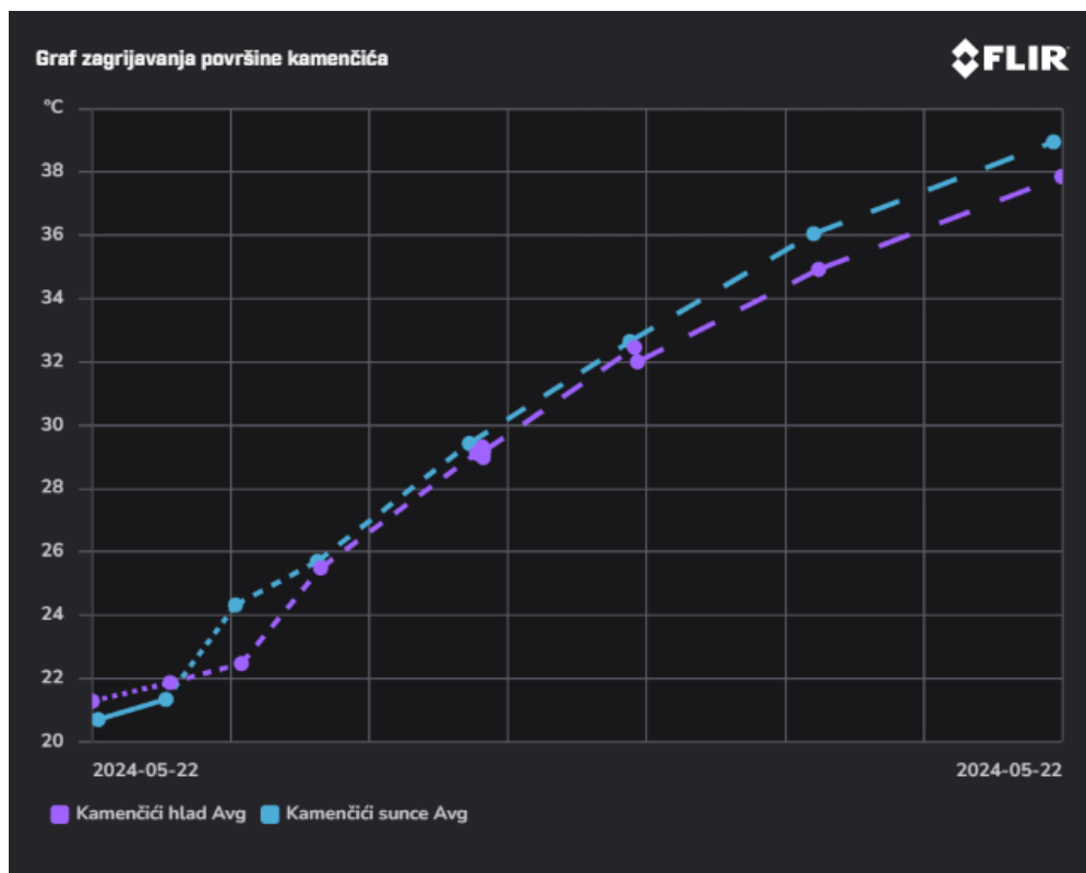
Slika 4.6: Usporedba temperatura površine kamenčica pod suncem i u hladu
