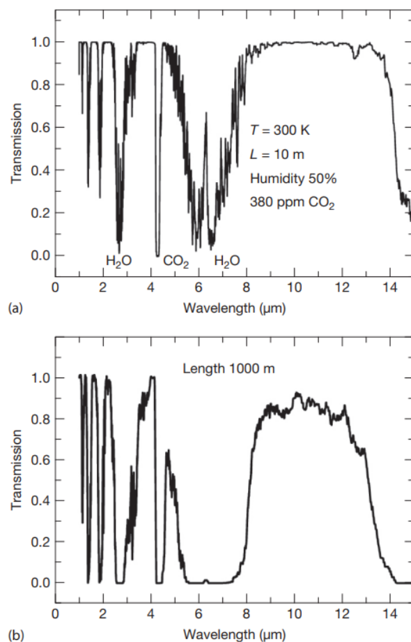
Slika 2.2: Transmisija infracrvenog zračenja kroz atmosferu u ovisnosti o valnoj dužini, izvor: Vollmer M., Möllmann K.-P. Infrared Thermal Imaging, Second Edition, poglavlje 1
