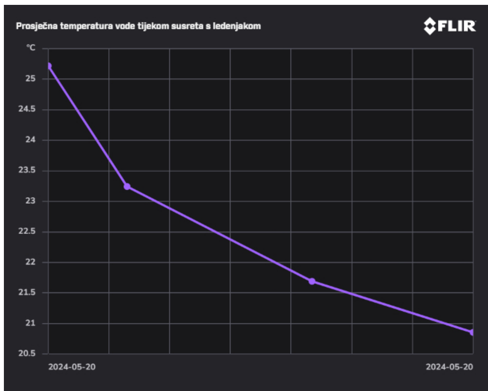
Slika 4.15: Promjena prosječne temperature vode tijekom pokusa
