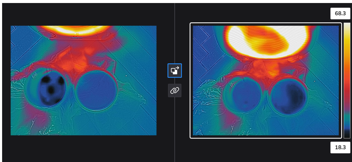
Slika 4.17: Pokus 3: Endotermna reakcija otapanja šumećih tableta
