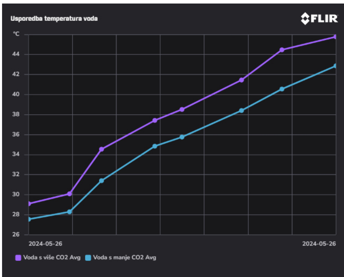
Slika 4.20: Pokus 3: Usporedba porasta prosječnih temperatura voda
