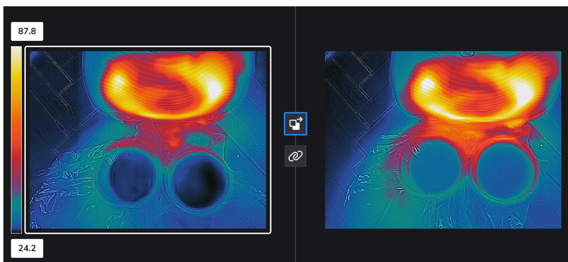
Slika 4.18: Postav 3: površinska temperatura voda se nakon nekog vremena izjednačava
