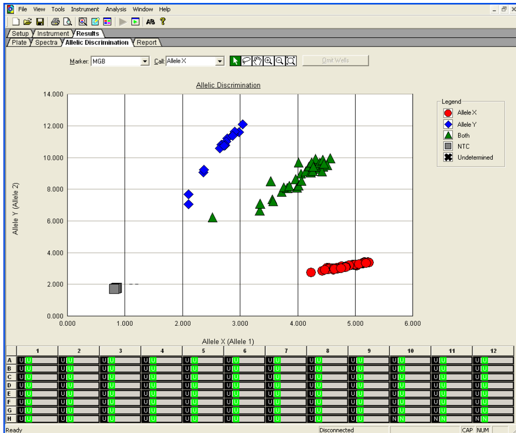
Slika 9. Alelna diskriminacija.
