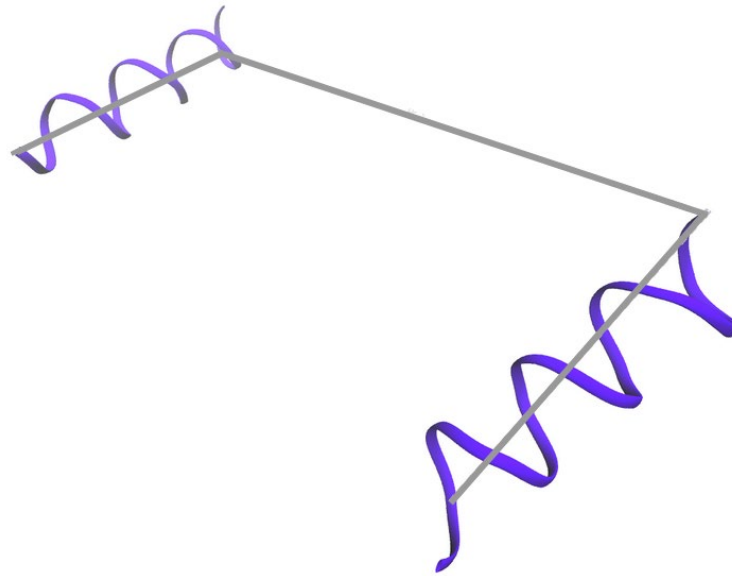
Slika P1. Grafički prikaz definicije dihedrnog kuta između DNA-vezujućih zavojnica. Zavojnice su definirane aminokiselinskim ostacima rednih brojeva od 46 do 58. Vizualizacija je dobivena pomoću programa VMD .
