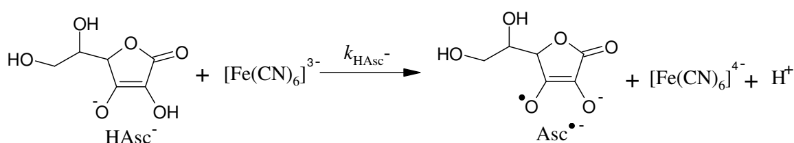
Shema 2.1. Prvi reakcijski stupanj u reakciji oksidacije askorbata heksacijanoferrat(III) ionom. Preuzeto iz reference 43.
