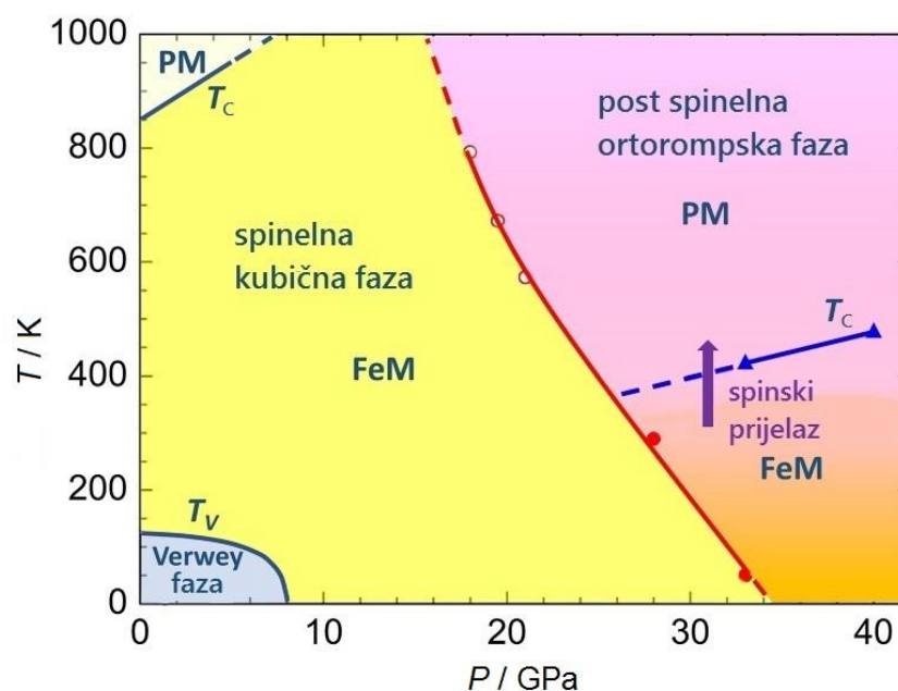
Slika 2.40. P-T fazni dijagram \text{Fe}_3\text{O}_4 uz naznačene granice faza; PM – paramagnetična, FeM – feromagnetna faza, T_C – Curieva temperatura, T_V – Verweyeva temperatura [597].
