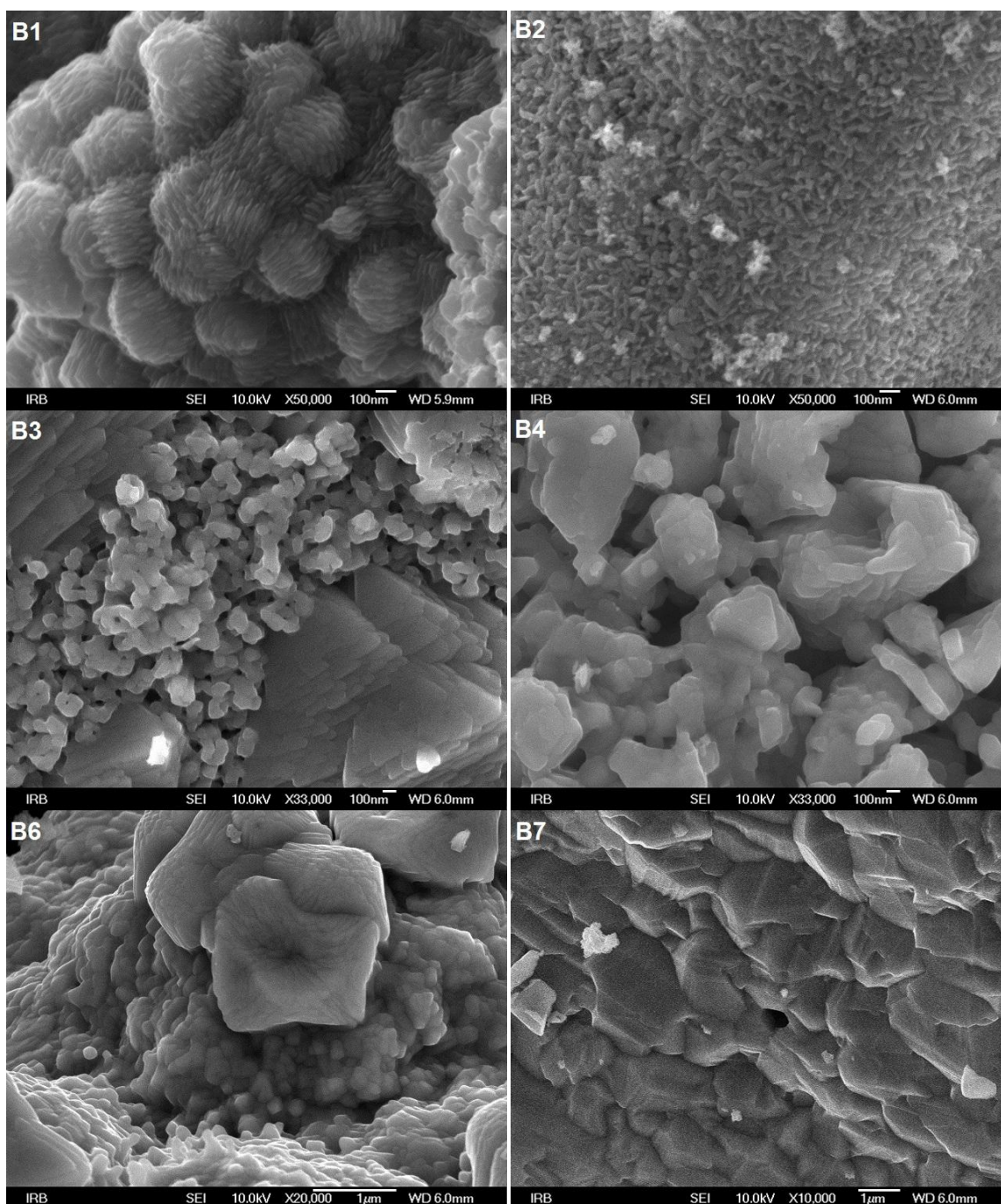
Slika 5.8. FE SEM mikrografije uzorka manganovih oksida nastalih termičkim raspadom Mn(NO_3)_2 \cdot xH_2O .
