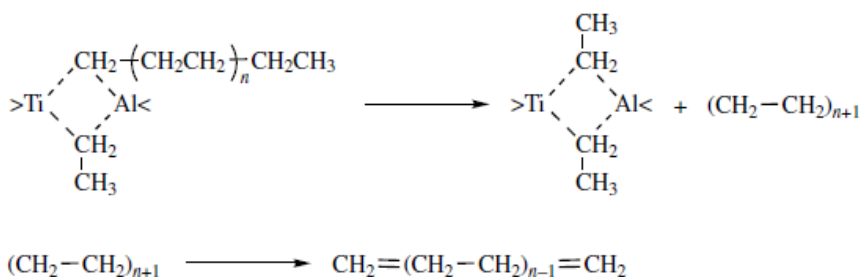
Slika 3: prikaz načina rada katalizatora TiCl_3 pri koordinacijskoj polimerizaciji u stupnjevima inicijacije, propagacije i terminacije lanca
