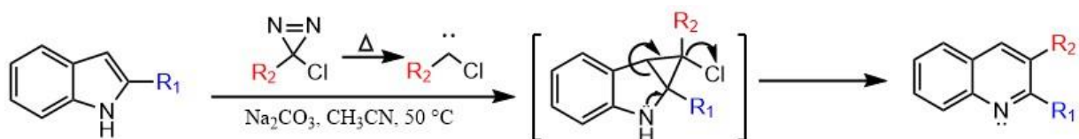
Slika 8. Sintaza kinolinskog produkta iz supstituiranog indola. 12
