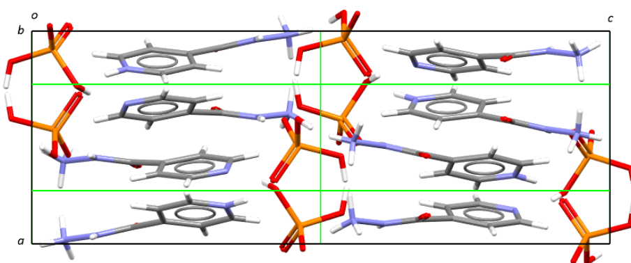
Slika D44. Projekcija kristalne strukture soli (HINZ)(H 2 PO 4 ) duž kristalografske osi b .
