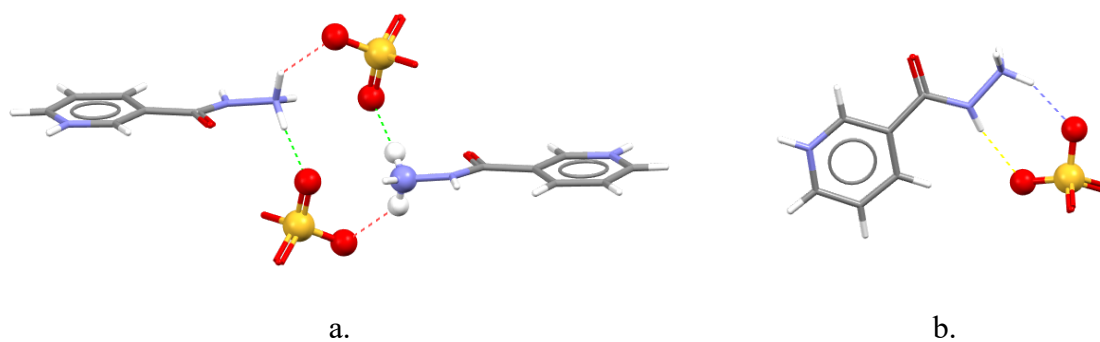
Slika D48. Graf-set oznake prstenastih sintona unutar kristalne strukture (H_2NZ)SO_4 :
