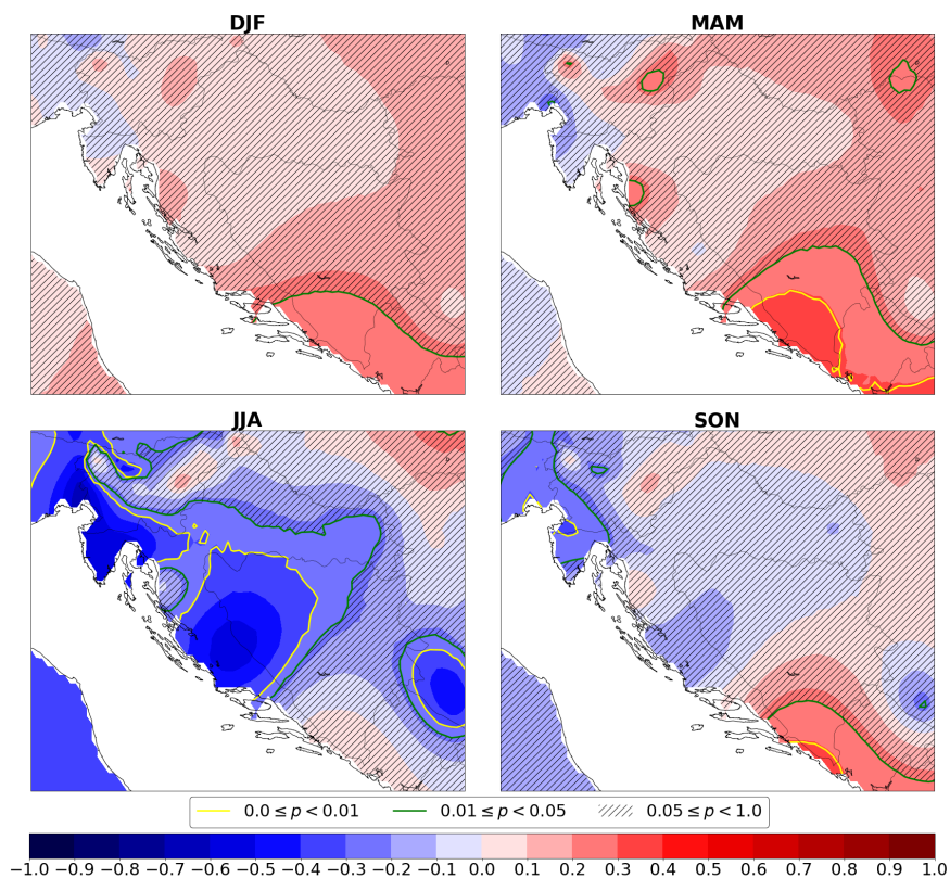
Slika 3.6 Sezonske korelacijske mape SLP-a i EAI-a za svaku sezonu s izolinijama p-vrijednosti koje označavaju statističku značajnost polja korelacijskih vrijednosti.
