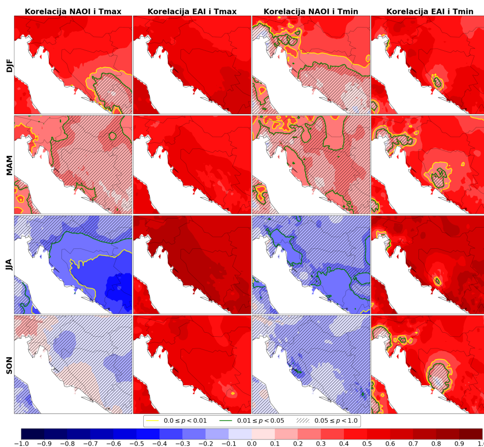
Slika 3.11 Sezonske korelacijske mapе ekstremnih temperatura i modova klimatske varijabilnosti s izolinijama koje prikazuju statističku značajnost koeficijenata korelacije.
