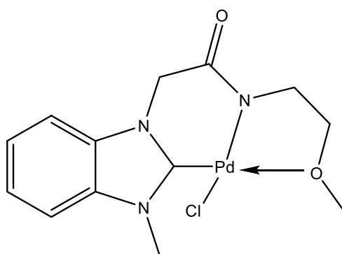
Slika 13. Struktura Pd (II) NHC-amidatnog-alkoksidnog kompleksa ( 28 ) 13(b)
