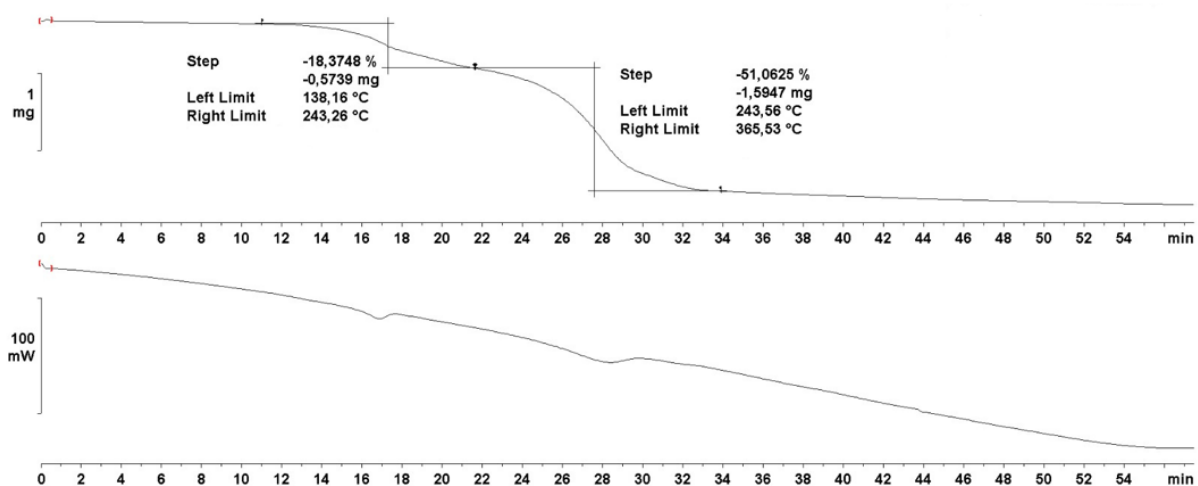
Slika D23. TG i DSC krivulje (rac-DAP)[CuCl_4]
