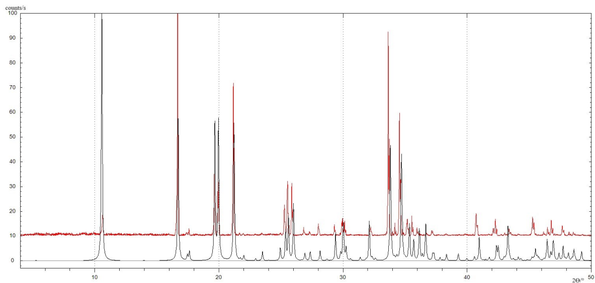
Slika D1. Usporedba difraktograma praha (rac-DAP)[CuCl_4] priređenog otopinskom sintezom (crveno) i simuliranog difraktograma praha (rac-DAP)[CuCl_4] izračunatog na temelju podataka difrakcije rendgenskih zraka na jediničnom kristalu (crno)
