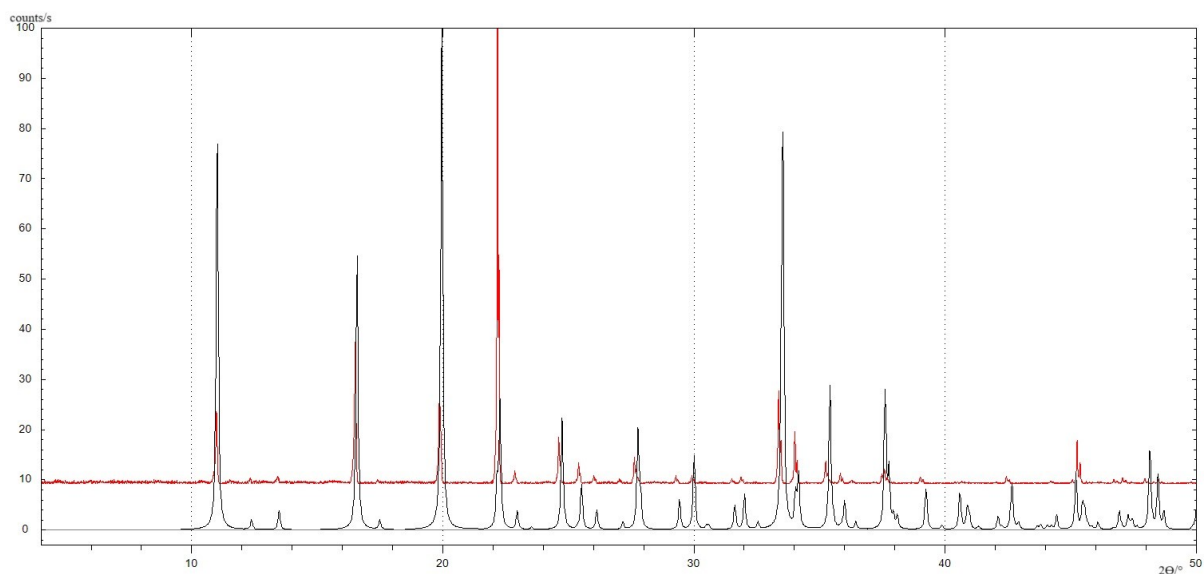
Slika D2. Usporedba difraktograma praha (R-DAP)[CuCl_4] priređenog otopinskom sintezom (crveno) i simuliranog difraktograma praha (R-DAP)[CuCl_4] izračunatog na temelju podataka difrakcije rendgenskih zraka na jediničnom kristalu (crno)
