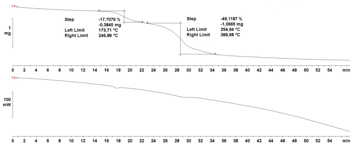
Slika D24. TG i DSC krivulje (R-DAP)[CuCl_4]
