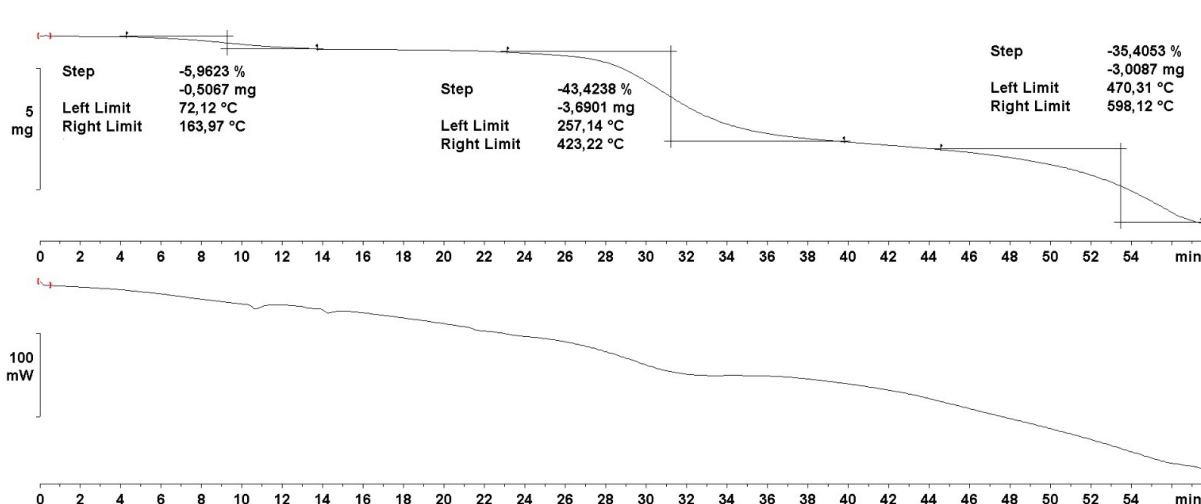
Slika D31. TG i DSC krivulje R-(DAP)[ZnCl_4] \cdot H_2O
