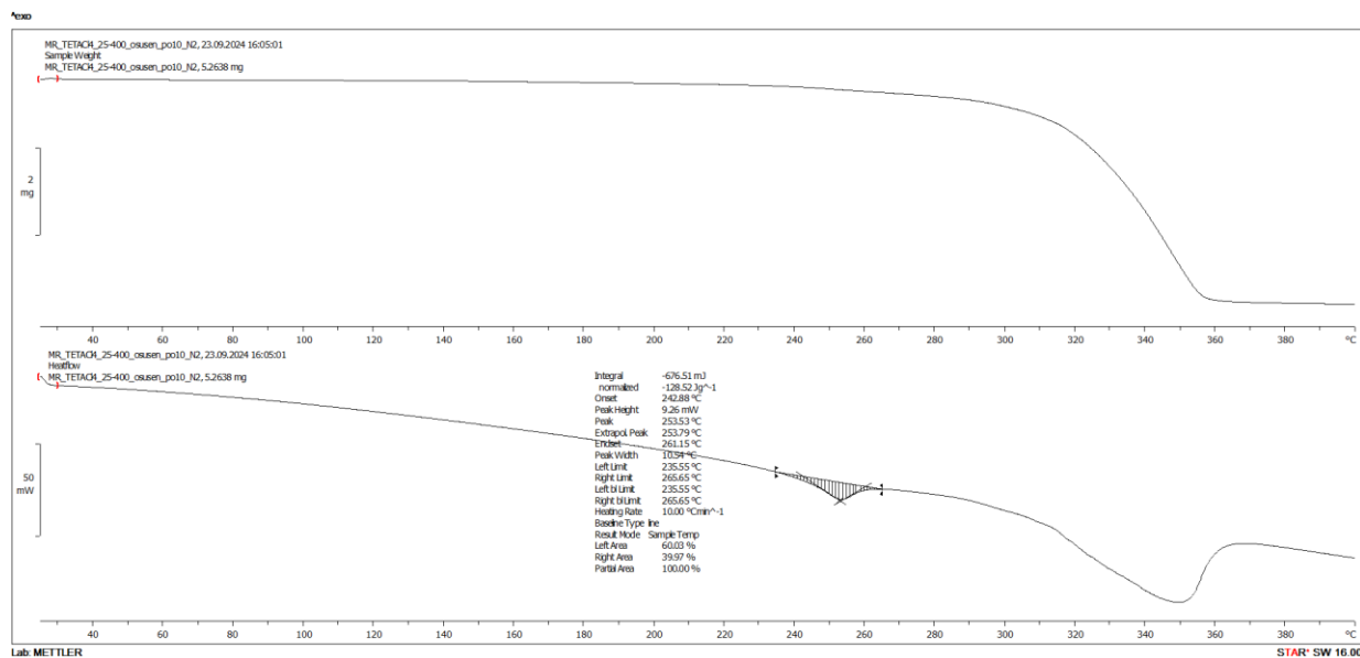
Slika D13. TG/DSC krivulja pripravljene kloridne soli trietilentetraamina: (\text{H}_4\text{TETA})\text{Cl}_4 .
