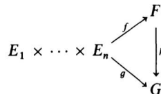
Slika 0.1: Dijagram tenzorskog produkta; slika iz [3]
