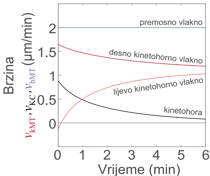
Slika 3.4: Rezultati modela koji pokazuju promjene u vremenu brzina kinetohora (crno), kinetohornih vlakana (crveno) i premosnih vlakana (plavo) za kinetohore početno izmaknute 2 \mu\text{m} lijevo od središta diobenog vretena. Svi parametri su kao u tablicama 3.1 i 3.2. Slika je adaptirana iz [84].
