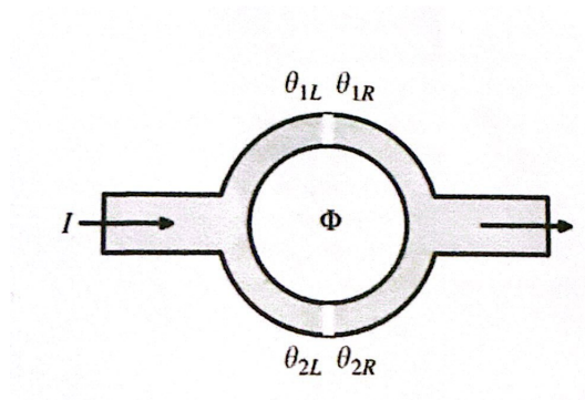
Slika 5.3: Shematski prikaz SQUID-a, preuzeto iz [1], str. 118.
