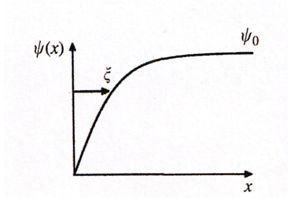
Slika 3.1: Prostorna ovisnost parametra uređenja s označenom skalom duljine koherencije, preuzeto iz [1] str. 76.
