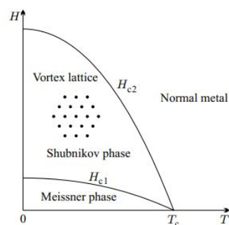
Slika 2.4: Fazni dijagram supravodiča tipa II, preuzeto iz [2], str. 457
