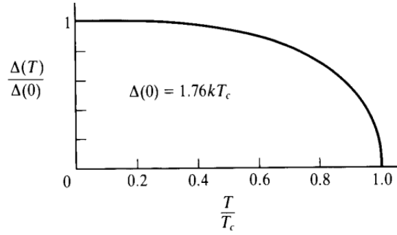
Slika 4.4: Temperaturna ovisnost procijepa u BCS teoriji, preuzeto iz [5], str. 64.
