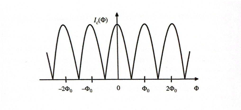
Slika 5.4: Ovisnost kritične struje o magnetskom toku, preuzeto iz [1], str. 120.
