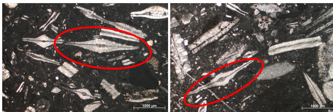
Slika 16 Fotomikrografije mikroskopskih preparata s osnim presjecima ortofragmina prepoznatih kao predstavnici morfogrupe Discocyclina augustae WEIJDEN (uzorak ZM2a).
