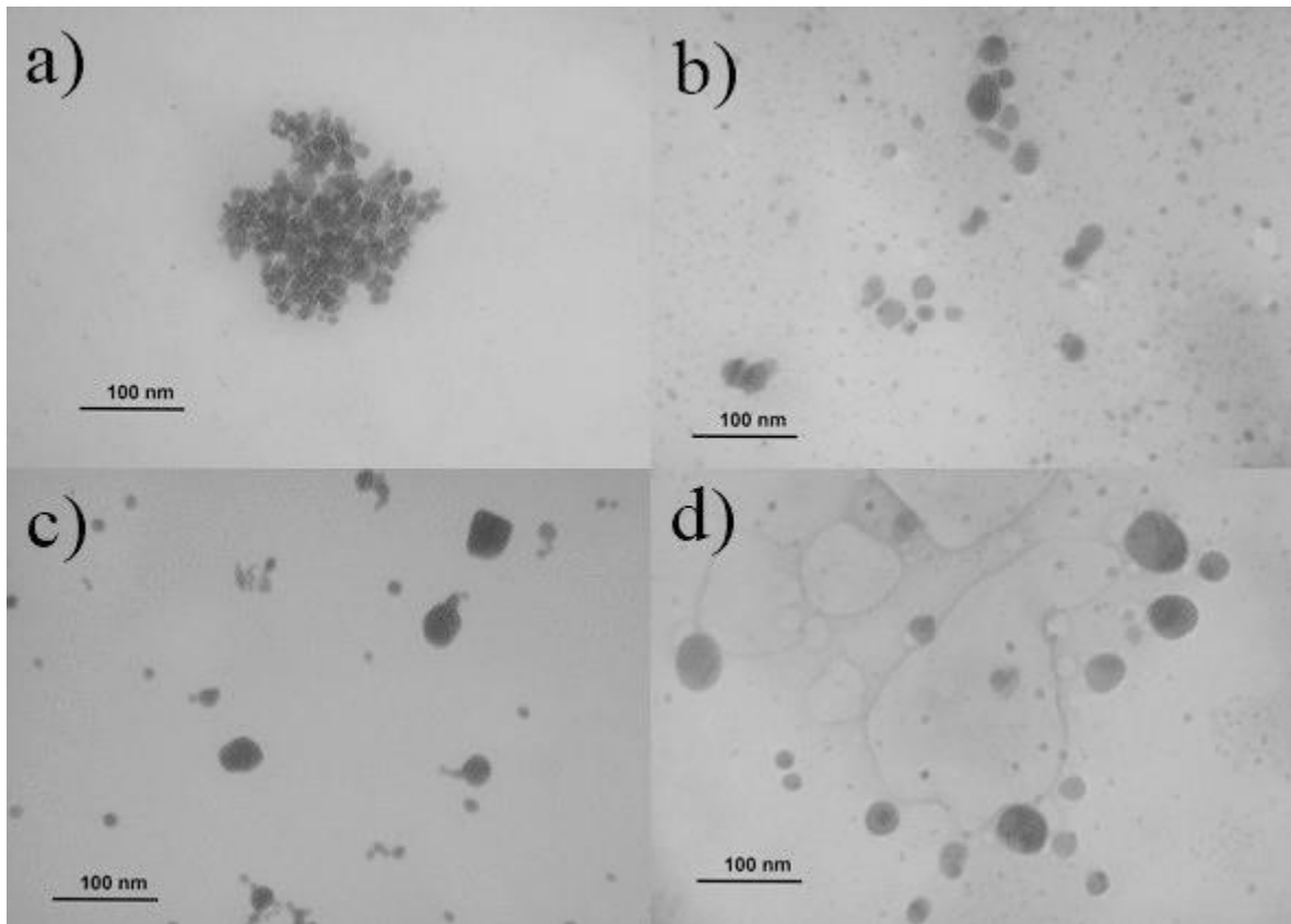
Slika 17. TEM fotografije korištenih nanočestica zlata i srebra: a) CYSnanoAg, b) GSHnanoAg, c) CYSnanoAu, d) GSHnanoAu (preuzeto iz Ivanković, 2016).
