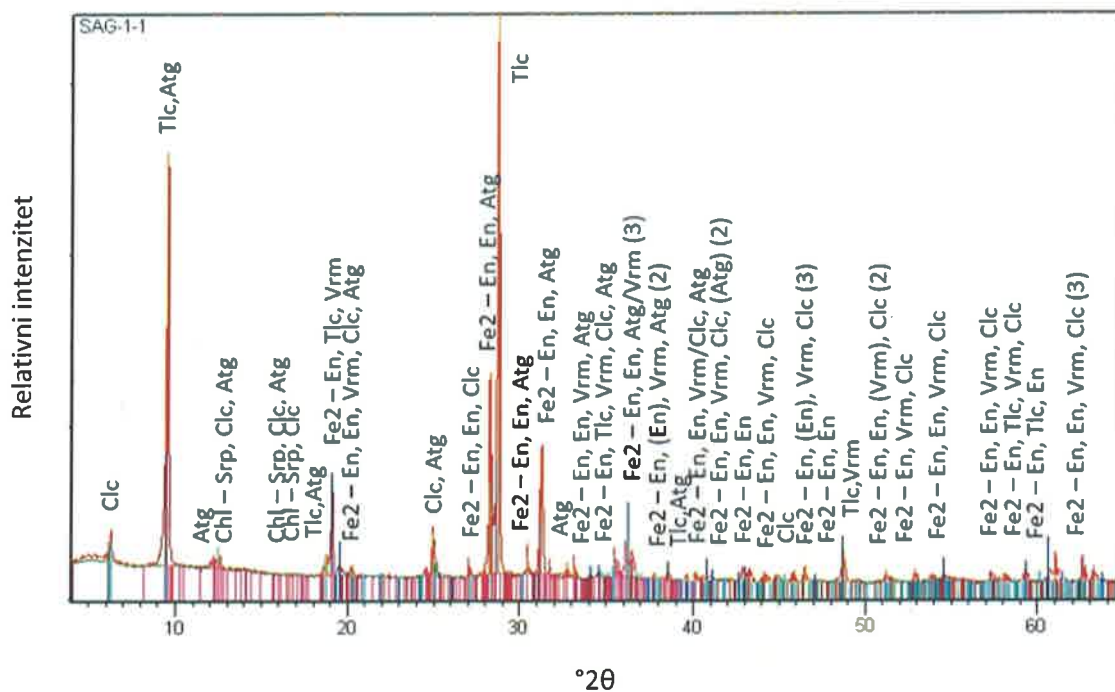
Slika 32. Difraktogram uzorka SAG 1.1 (Clc – klinklor, Tlc – talk, Atg – antigorit, Chl-Srp – klorit-serpentin, Fe2-En – željezoviti enstatit/bronicit, En – enstatit, Vrm – vermikulit)
