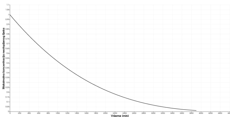
Slika 4.2: Maksimalna koncentracija neotopljenog lijeka po elementima \max_{\mathbf{x} \in \Omega} s(t, \mathbf{x}) tijekom 60 sati
