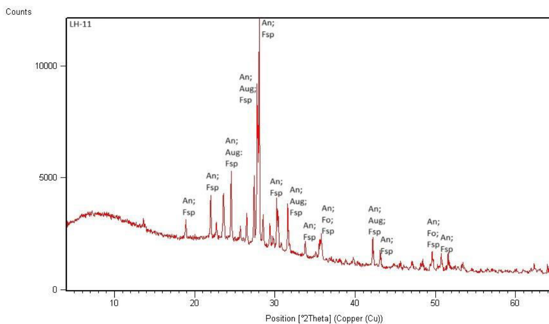
Slika (18) – Difraktogram uzorka LH-11. Uzorak sadrži: Anortit (An), Augit (Aug), Forsterit (Fo) i Feldspat (Fsp). Kratice minerala prema (Whitney & Evans, 2010).
