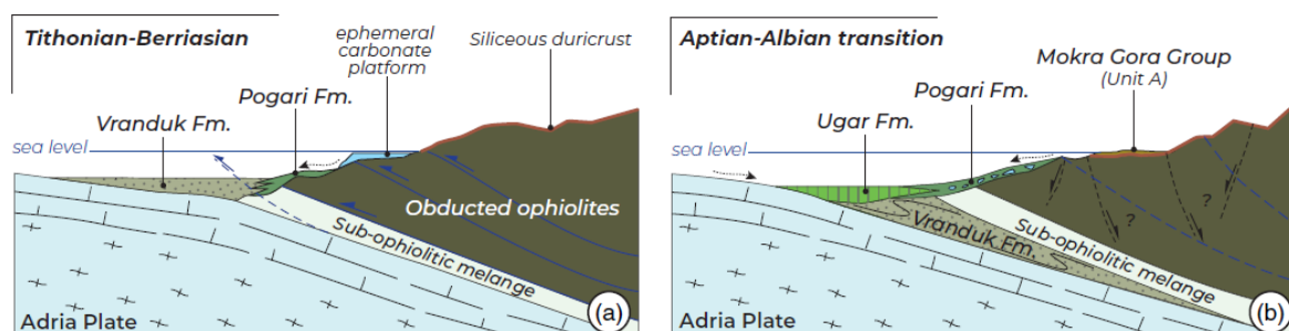
Slika 5. Razvoj Vrandučke i Ugar formacije zajedno s prikazom paleogeografije u to vrijeme. (a) početak taloženja Vrandučkog fliša na granici jura/kreda (titi – berijas). Vidljivo je da je tada obdukcija ofiolita Zapadnovardarske zone bila završila. Crna, isprekidana strijelica prikazuje smjer paleotransporta. U slučaju Vrandučkog fliša smjer paleotransporta bio je prema istoku, odnosno izvor detritusa bile su ofiolitne, bazične ili ultrabazične stijene (b) početak taloženja Ugar formacije u krovini Vrandučke formacije na granici apt – alb u donjoj kredi. Smjer paleotransporta za Ugar formaciju bio je prema sjeveroistoku, odnosno izvorne stijene bili su plitkomorski karbonati Jadranske karbonatne platforme (modificirano prema NIRTA i sur., 2020)
