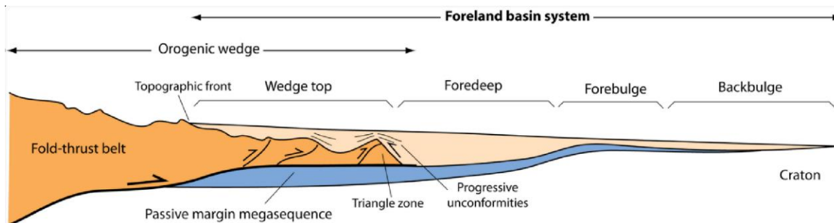
Slika 1. Shematski prikaz sustava predgorskog bazena sa sedimentacijskim zonama (prema DECELLIES i GILES, 1996)
