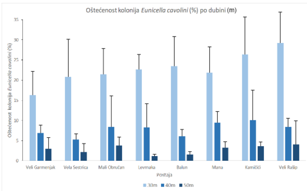
Slika 28. Oštećenost kolonija žute rožnjače Eunicella cavolini na istraživanim postajama po dubinama (prosječan broj oštećenih kolonija za 2012., 2022. i 2023. godinu \pm SD).
