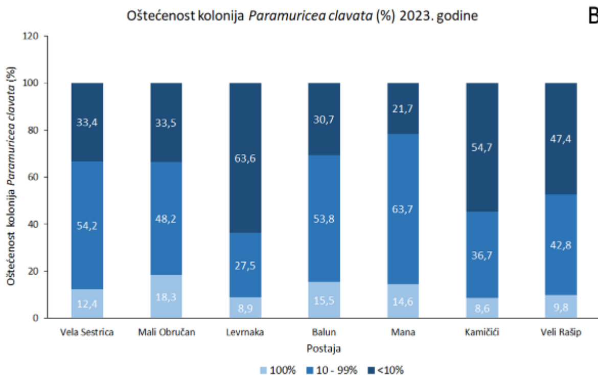
Slika 35. Oštećenost crvene rožnjače Paramuricea clavata na istraživanim postajama (prosječan broj oštećenih kolonija \pm SD). A) ukupno oštećenih kolonija; B) postoci oštećenih kolonija (<10% oštećenja), zahvaćenih kolonija (između \geq 10% i \leq 99% oštećenja) i mrtvih kolonija (100% oštećenja).
