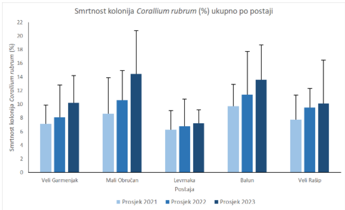
Slika 44. Smrtnost kolonija crvenog koralja Corallium rubrum na istraživanim postajama (prosječan broj uginulih kolonija \pm SD).
