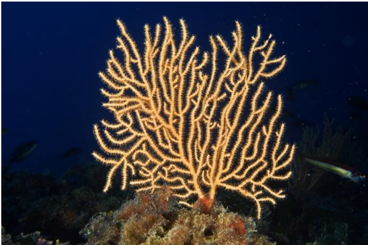
Slika 4. Kolonija vrste Eunicella cavolini . (P. Kružić)
