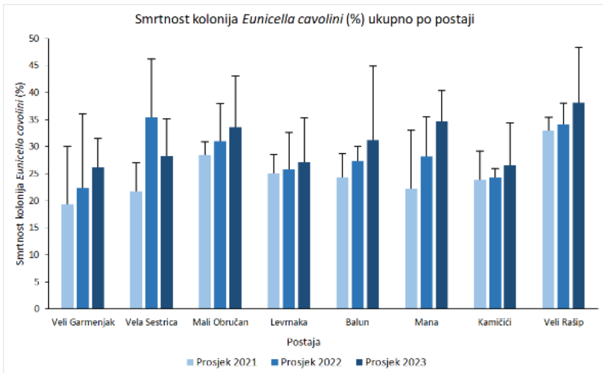
Slika 29. Smrtnost kolonija žute rožnjače Eunicella cavolini na istraživanim postajama (prosječan broj uginulih kolonija \pm SD).
