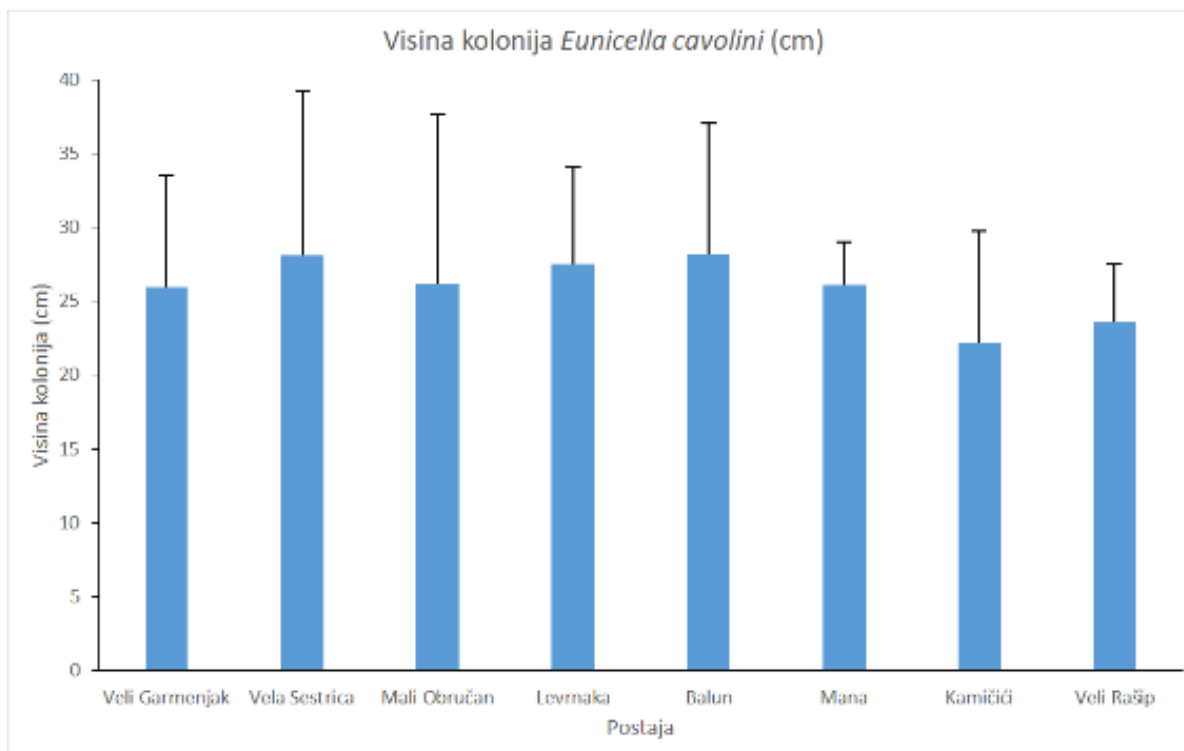
Slika 25. Visina kolonija vrste Eunicella cavolini na istraživanim postajama (prosjek \pm SD).
