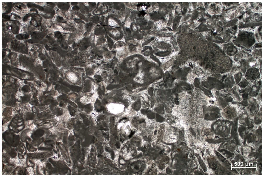
Slika 7: Litoklastično-bioklastični packstone – grainstone / grainstone, mikroskopski preparat TS-6/2.
