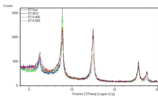
Usporedni rendgenogram orijentiranih preparata uzorka ET-5.
