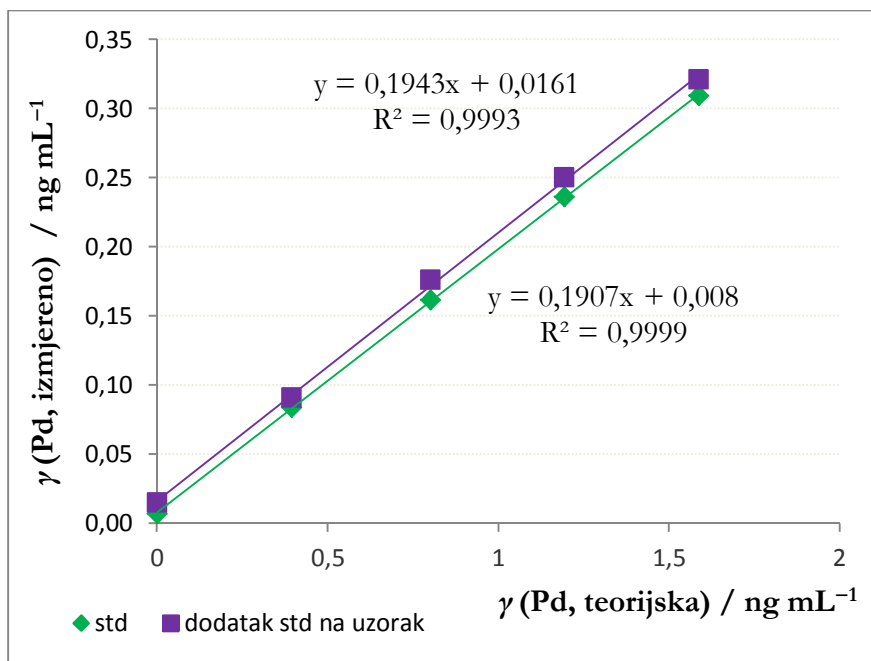
Slika 24. Odnos izmjerenih i teorijskih vrijednosti paladija u pročišćenom uzorku BCR 723 nakon dodatka smjese standarda PGE
