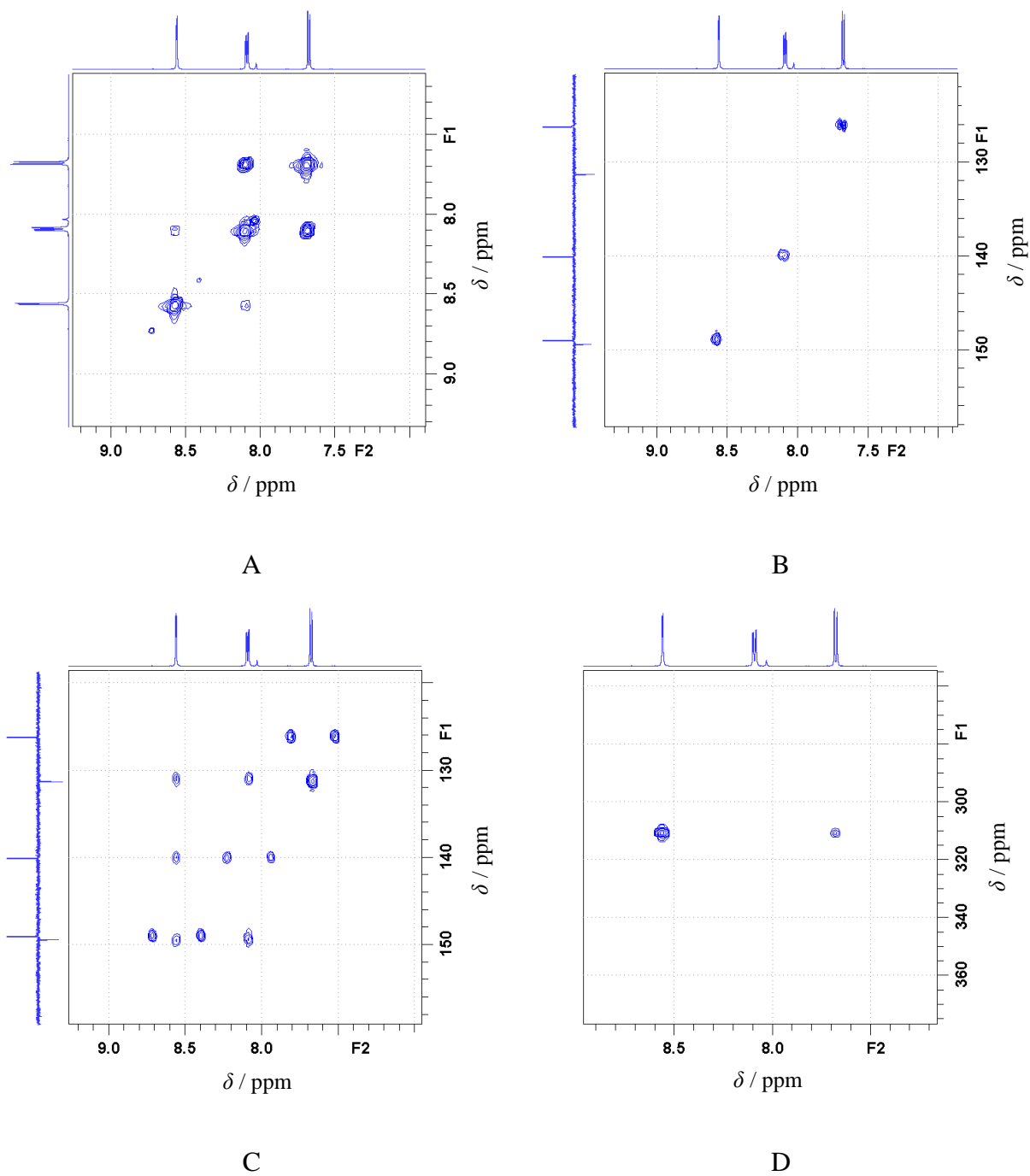
Slika D57. Uvećani prikaz A) ^1H-^1H COSY, B) ^1H-^{13}C HMQC, C) ^1H-^{13}C HMBC i D) ^1H-^{15}N HMBC spektara NMR kompleksa [Ag(NO_3)(2,5-Cl_2py)_2] , ( K7 ).
