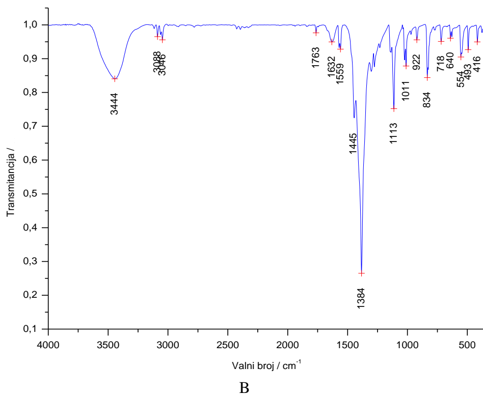
Slika D24. Spektri IR A) 2,5-Cl 2 py (L7) i B) [Ag(NO 3 )(2,5-Cl 2 py) 2 ] (K7).
