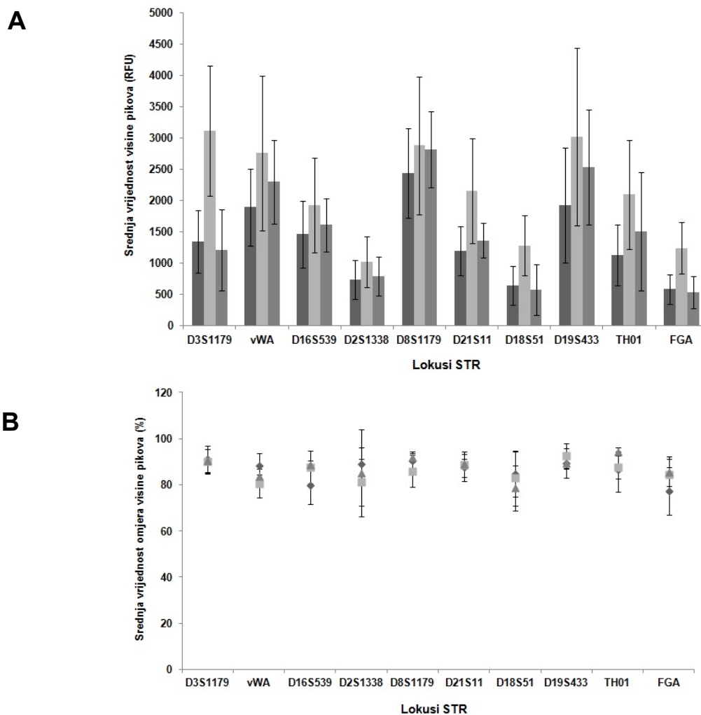
Slika 27. Visine pikova (RFU) i omjeri visina pikova (%) za uzorke krvi na drvu kao podlozi
