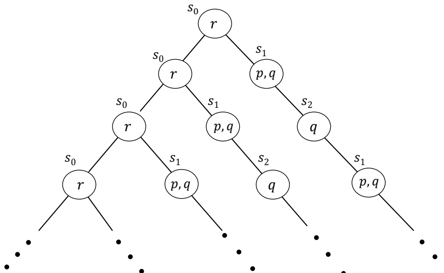
SLIKA 1.2: BESKONAČNO STABLO KOJE PRIKAZUJE SVE PUTEVE IZ STANJA s_0 MODELA ZADANOG SLIKOM 1
