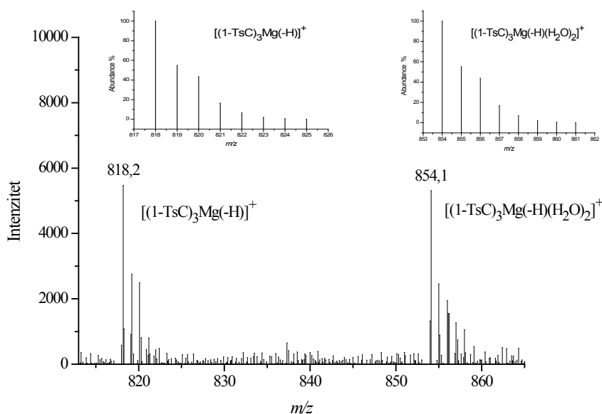
Slika 56: Razvučeni cjeloviti spektar, snimljen u ES^+ načinu rada, za signale na m/z 818,2 koji je asigniran kao [(1-TsC)_3Mg(-H)]^+ i na m/z 854,1 koji je asigniran kao [(1-TsC)_3Mg(-H)(H_2O)_2]^+ u uzorku (ligand 2 i Mg^{2+} ) u otapalu DMSO/MeOH (1/100), uz c=10^{-5} mol dm^{-3} te snimljen na spektrometru Agilent 6410 QQQ.
