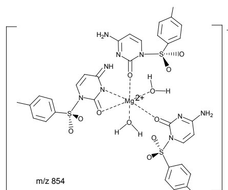
Slika 57: Prikaz moguće strukture za ion na m/z 854,1 assigniranog kao [(1\text{-TsC})_3\text{Mg}(-\text{H})(\text{H}_2\text{O})_2]^+ .
