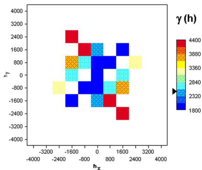
Slika 7.12. Karta variogramske površine za varijablu „ostatci“ polja Šandrovac
