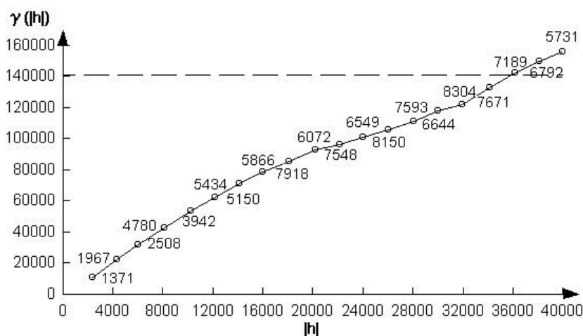
Slika 8.26. Ekperimentalni variogram glavne osi za varijablu „dubina“ po plohi EK markera \Delta
