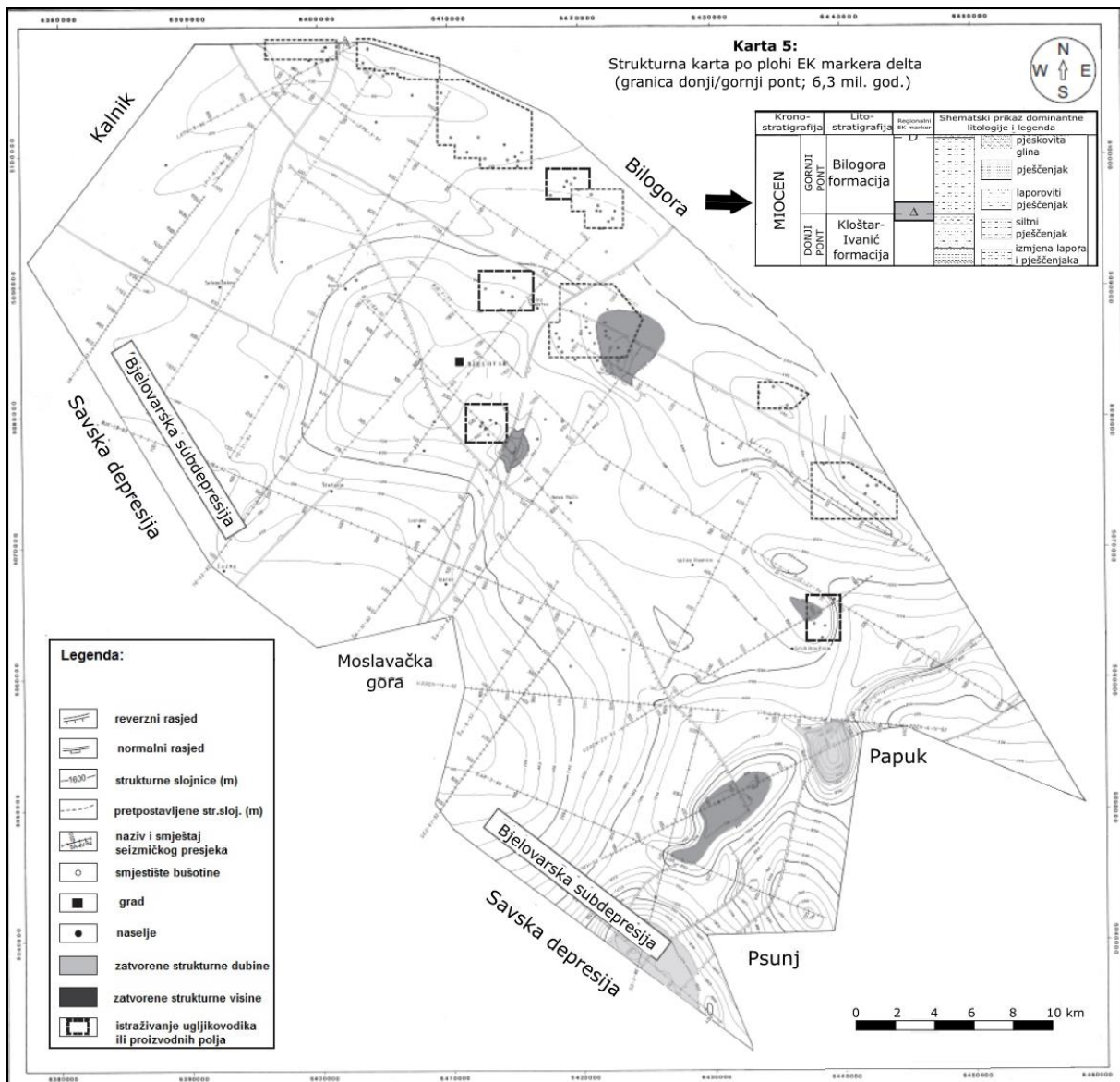
Slika 4.8. Strukturalna karta Bjelovarske subdepresije po plohi EK markera Δ (Malvić, 2011)
