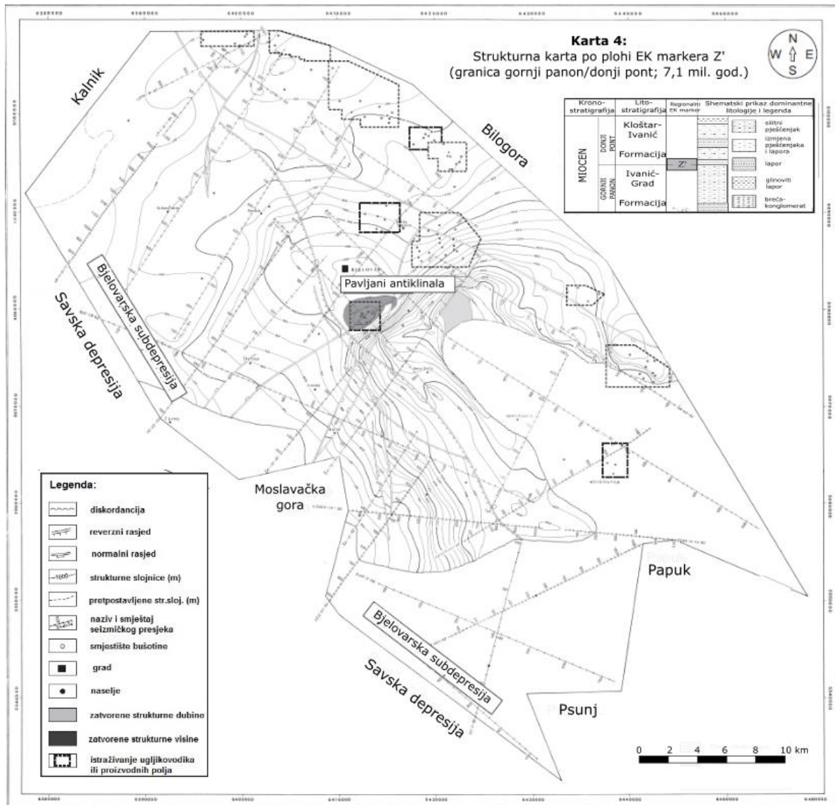
Slika 4.7. Strukturalna karta Bjelovarske subdepresije po plohi EK markera Z' (Malvić, 2011)
