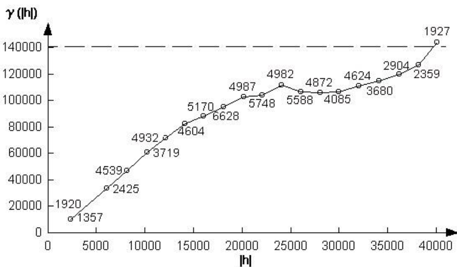
Slika 8.27. Ekperimentalni variogram sporedne osi za varijablu „dubina“ po plohi EK markera \Delta
