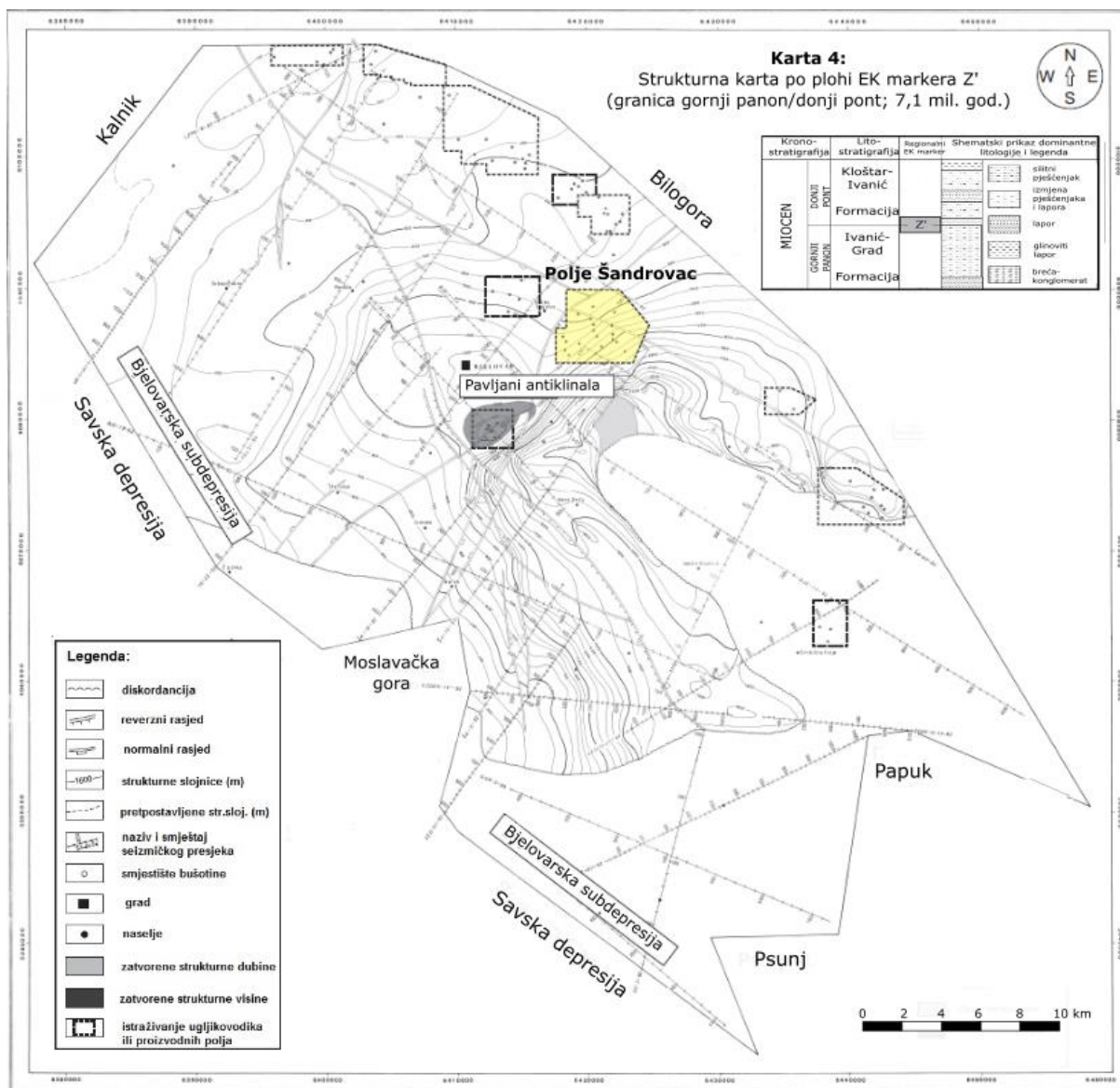
Slika 7.2. Strukturalna karta Bjelovarske subdepresije po plohi EK markera Z' (Malvić, 2011) i položaj polja Šandrovac
