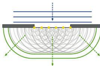
Slika 2.22. Huygensov princip na pukotini.
