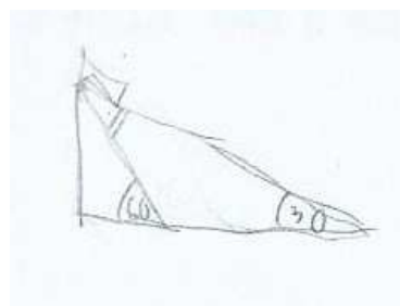
Slika 31. Različite vizualizacije fizikalne situacije u šestom zadatku.
