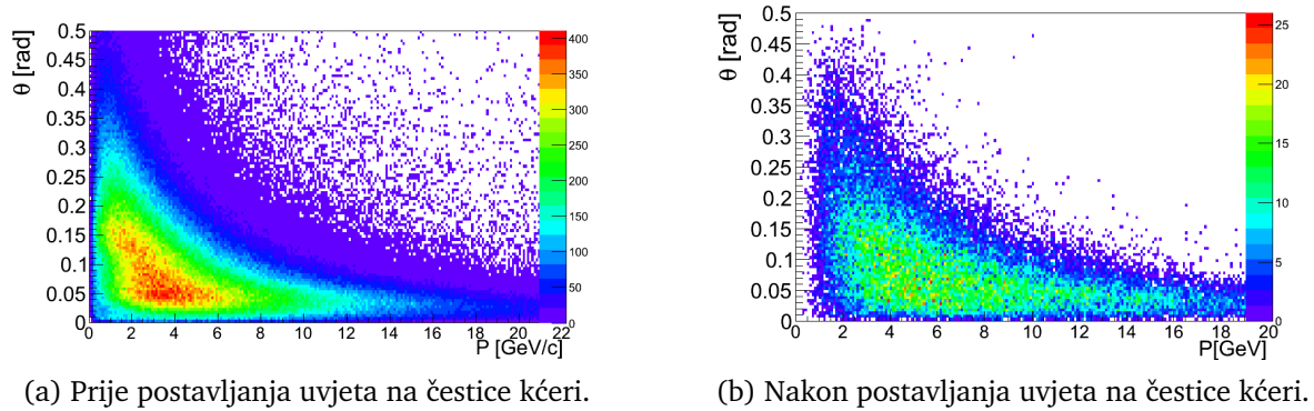
Slika 3.11: Broj V^0 kandidata u ovisnosti o ukupnom impulsu p i polarnom kutu \theta za TI uzorak.
