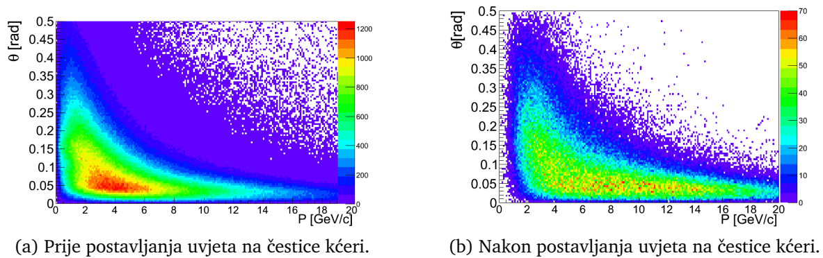
Slika 3.12: Broj V^0 kandidata u ovisnosti o ukupnom impulsu p i polarnom kutu \theta za MC uzorak.
