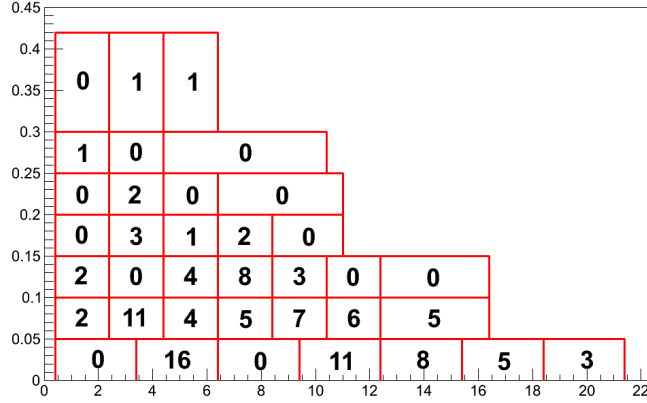
Slika 3.18: Broj \Lambda hiperona u p - \theta intervalima u TR uzorku.
