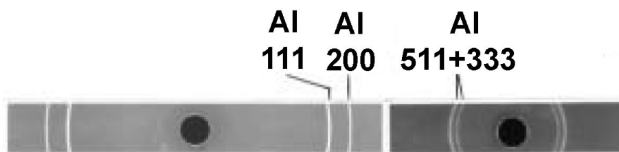
Slika 3.5: Slika dobivena Debye-Scherrerovom kamerom. Uzorak: popuštani čisti aluminijski
