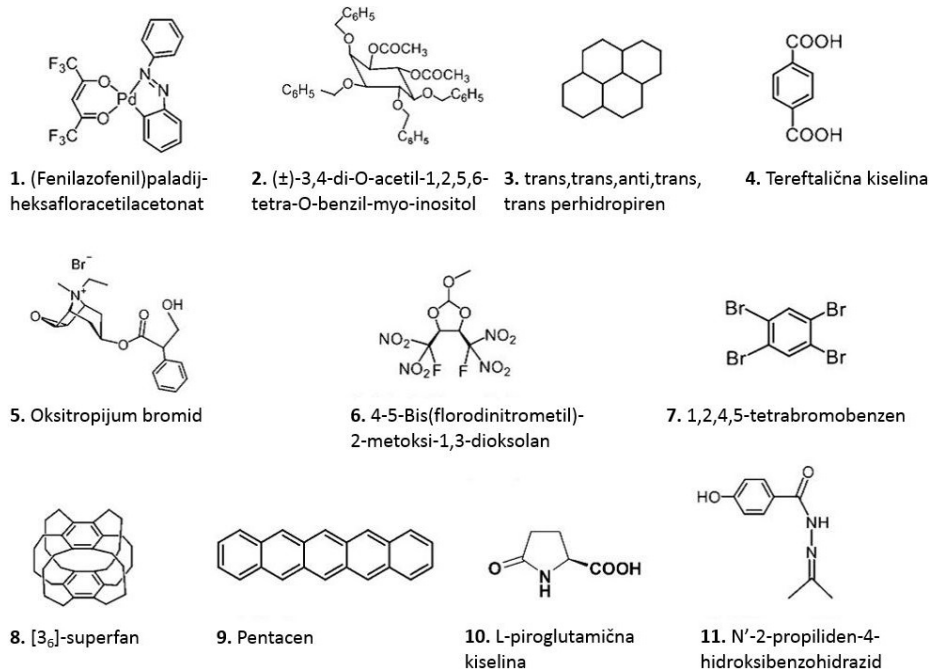
Slika 2.1: 11 kemijskih spojeva kod kojih je dosad uočen termosolientni efekt
