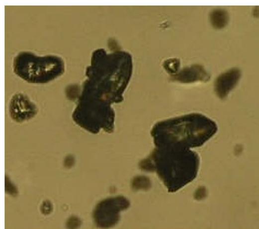
Slika 4.11: Kristali prije (lijevo) i poslije (desno) faznog prijelaza III \rightarrow II na temperaturi od 88 °C
