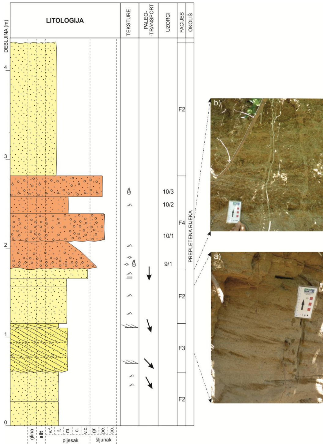
Prilog 1.8. Sedimentološki stup Petravec-I (Pet-I); a) Prikaz setova kose tangencijalne slojevitosti u srednjezrnatim pijescima facijesa F3 (uz gornji rub mjerilice nalazi se ravna oštra granica prema srednjezrnatim pijescima facijesa F2); b) Pjeskoviti šljunci facijesa F4 čija se donja erozijska granica nalazi u razini mjerilice.
