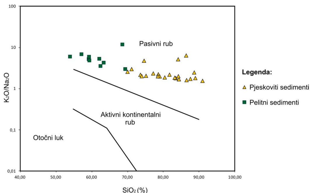
Slika 5.16. Tektoski diskriminantni dijagram na osnovi odnosa K 2 O/Na 2 O i SiO 2 (wt%) (prema primjeru iz ROSER i KORSCH, 1986) za pjeskovite i pelitne sedimente Viviparus slojeva s područja Vukomeričkih gorica.
