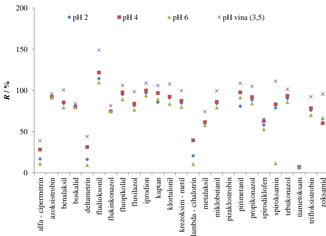
Slika 32. Optimizacija SPE – ovisnost analitičkog povrata ( R ) pesticida iz crnog vina o pH uzorka.
