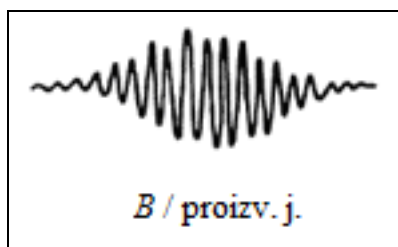
Slika 44: EPR spektar tritilijevog radikala, nastalog u reakciji benzimidazolina LP 32 s trifenilklormetanom 156
