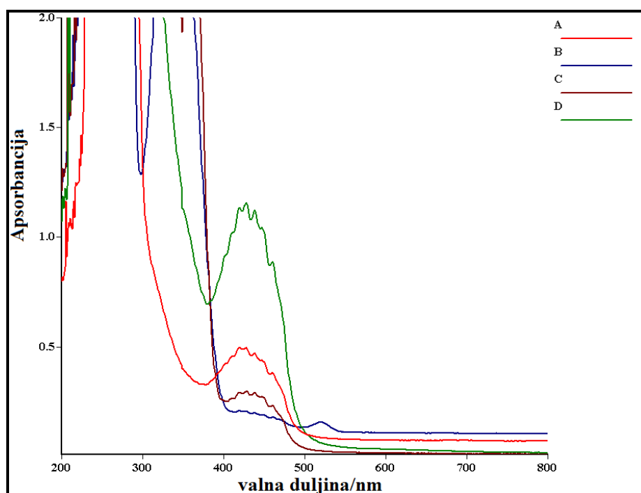
Slika 75: UV-Vis spektar:
