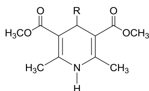
Tablica 17: Aromatizacija 2,6-dimetil-3,5-di(metoksikarbonil)-4-alkil-1,4-DHP s MoCl_5
