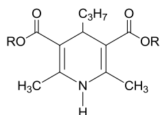
Tablica 20: Aromatizacija 2,6-dimetil-3,5-di(alkiloksikarbonil)-4-(prop-1-il)-1,4-DHP s \text{VOCl}_3
