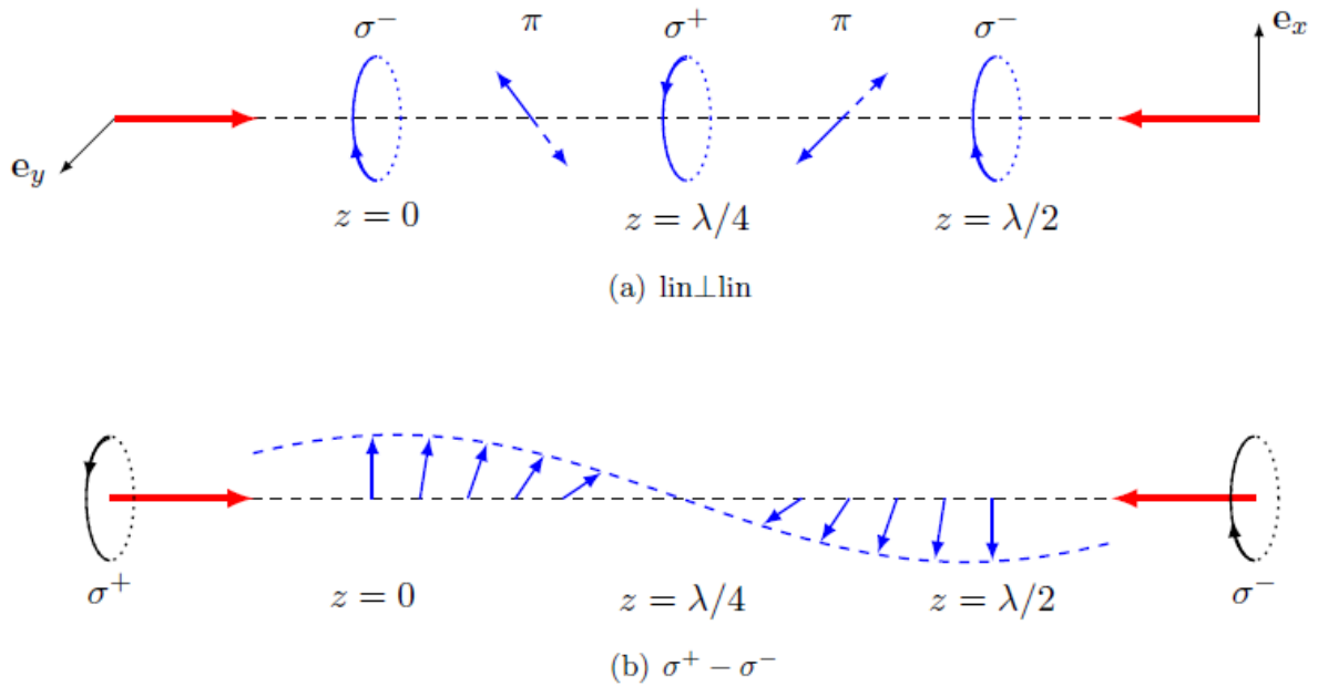
Slika 2.6: Dva tipa polarizacijskog gradijenta u 1D optičkim melasama ostvoreni a) \text{lin}\perp\text{lin} konfiguracijom i b) \sigma^+\sigma^- konfiguracijom. Preuzeto iz [18].
