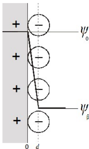
Slika 2. Model molekulskog kondenzatora.
