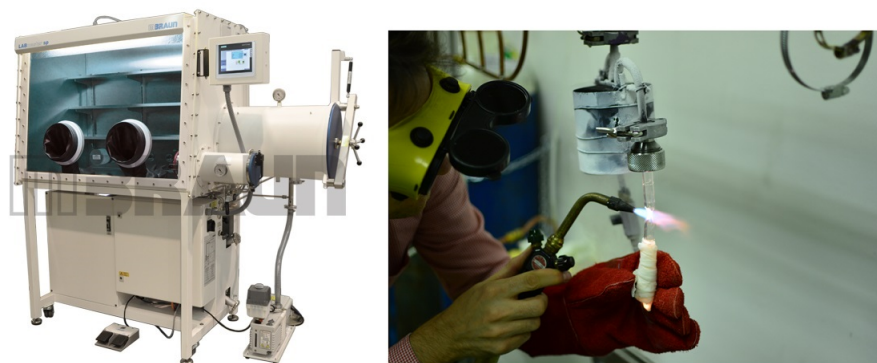
Slika 5.1: (lijevo) Glovebox komora korištena za miješanje elemenata za sintezu. (desno) Zatvaranje druge strane ampule nakon ispumpavanja.
