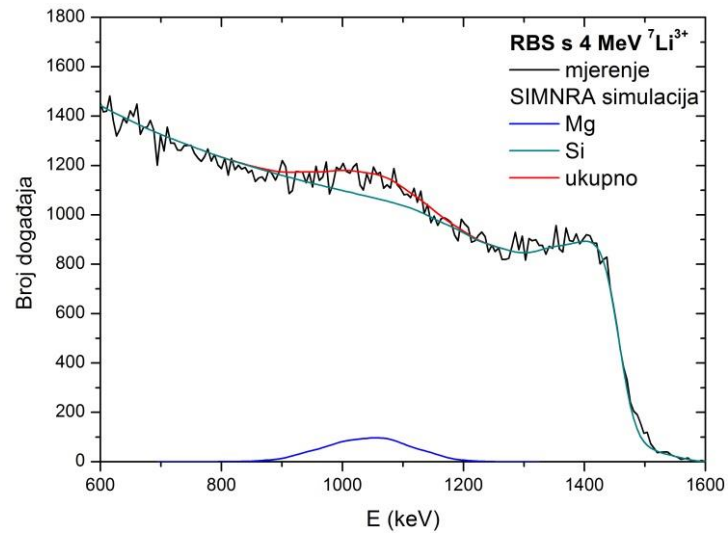
Slika 4.17. RBS spektr dobiven pomoću snopa 4 MeV-skih ^7\text{Li}^{3+} iona na uzorku Si implantiranog sa 180 keV-skim ^{24}\text{Mg} ionima (velika doza).
