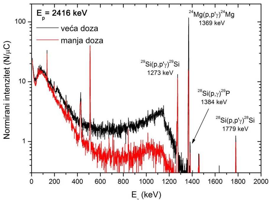
Slika 4.7. Usporedba gama-spektara Si uzorka implantiranih sa 180 keV-skim 24 Mg ionima s većom i manjom dozom dobiveni pobudom protonima energije 2416 keV-a.
