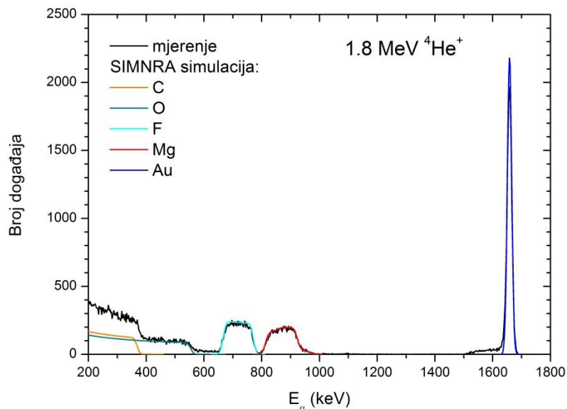
Slika 3.7. Spektar unatrag elastično raspršenih 1.8 \text{ MeV} -skih alfa-čestica na meti \text{MgF}_2 .
