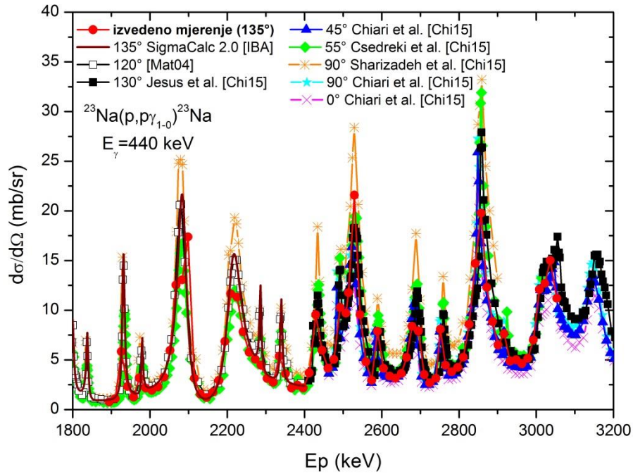
Slika 3.20. Usporedba izmjerenoeg diferencijalnog udarnog presjeka za produkciju gama-zračenja na 440 keV-a iz ^{23}\text{Na}(p,p'\gamma)^{23}\text{Na} reakcije s podacima naknadno dostupnim u bazi podataka [IBA] i uključenih u zajedničku publikaciju [Chi15] te evaluiranim diferencijalnim udarnim presjekom [Gur14].
