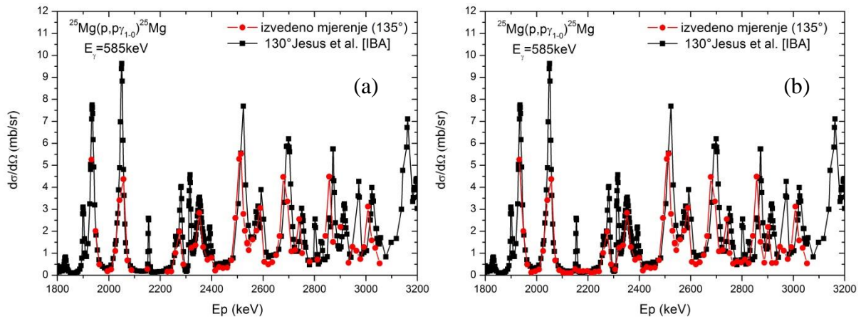
Slika 3.29. (a) Usporedba izmjerelog diferencijalnih udarnog presjeka za produkciju gama-zračenja na 585 keV-a s mjerenjem naknadno dostupnim u bazi podataka [IBA]. (b) Dodane su i MDL vrijednosti za pojedine energije protona radi bolje predodžbe slaganja podataka.
