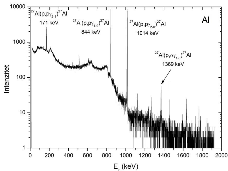
Slika 3.30. Gama-spekatar dobiven s Al mete pobuđene s protonima energije 2857 keV.
