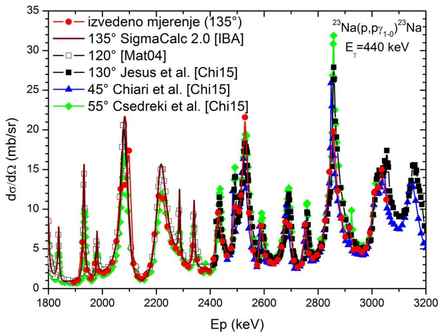
Slika 3.21. Usporedba izmjerenoeg diferencijalnog udarnog presjeka za produkciju gama-zračenja na 440 keV-a iz ^{23}\text{Na}(p,p'\gamma)^{23}\text{Na} reakcije s podacima naknadno dostupnim u bazi podataka [IBA] i uključenih u zajedničku publikaciju [Chi15] te evaluiranim diferencijalnim udarnim presjekom [Gur14] mjerenih na sličanom kutu.
