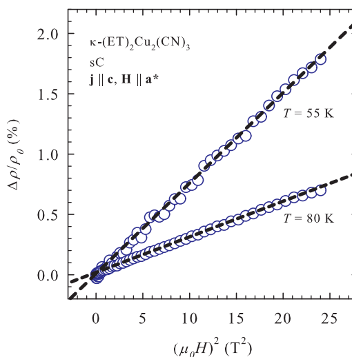
Slika 6.14: Ovisnost magnetootpora \kappa -(ET) 2 Cu 2 (CN) 3 (prazni plavi krugovi) iz serije sC mjenog u geometriji j || c , H || a * o kvadratu magnetskog polja na dvije reprezentativne temperature T = 55 \text{ K} i T = 80 \text{ K} . Crtkane crne linije predstavljaju prilagodbe na kvadratnu funkciju \Delta\rho/\rho_0 \sim H^2 .
