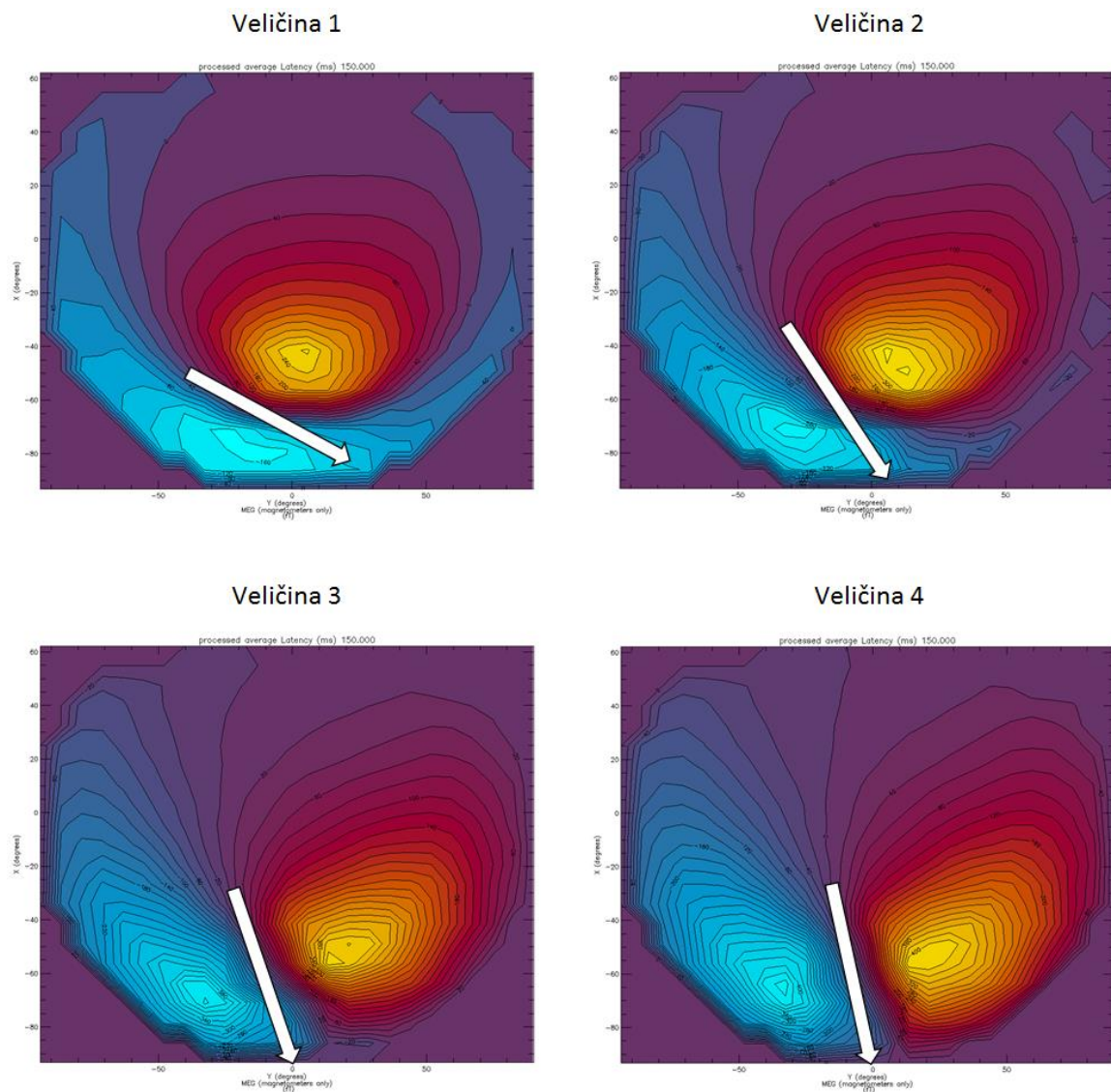
Slika•23. Horizontalna projekcija izoamplitudnih konturnih mapa simuliranog magnetskog polja na senzoriga za četiri rastuće veličine izvora na Lokaciji 1, u trenutku maksimuma aktivnosti, t = 150 ms. Strelica približno označava orijentaciju izvora.
