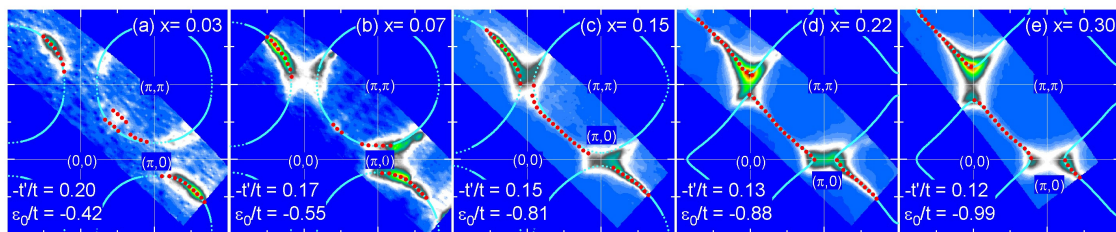
Slika 4.1: ARPES presjeci na Fermijevoj energiji za LSCO uzorke u širokom rasponu dopiranja [40]. Važno je primijetiti da se čak i u AF uzorcima s dopiranjem oko 1% primjećuje komad Fermijeve plohe. Duljina Fermijevog luka raste sa šupljinskim dopiranjem te oko vH dopiranja on seže u potpunosti do vH točke.
