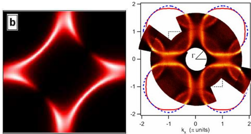
Slika 4.3: Fermijeve plohe jednoravninskog [42, 43] i toravninskog [44] Bizmutovog kuprata. Jednoravninski ima Fermijevu plohu sličnu LSCO-u, toravninski YBCO-u, s dugim ravnim dijelovima uz rub IBZ, sličnim 1D CDW sustavima. Iščezavanje Fermijevog luka na lijevoj slici je posljedica matričnog elementa foton-elektron vezanja, a ne pojava procjepa.
