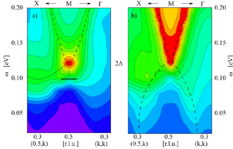
Slika 3.33: Učinak korelacija na niskotemperaturni magnetski spektar sa procjepom \Delta > 0 . Maximum na \mathbf{Q}_{AF} i \omega = 2\Delta te grana pobuđenja na frekvencijama iznad 2\Delta su vidljivi, ali se podigao intenzitet niskofrekvencijske nekomenzurabilne grane "pješčanog sata".
