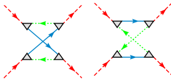
Slika 3.18: Dva doprinosa efektivnom međudjelovanju šupljina na jednoj bakrovoj orbitali, u formalizmu pomoćnih bozona i fermiona [29]. Crvene linije su metalne šupljine, a plave i zelene pomoni bozoni i fermioni.
