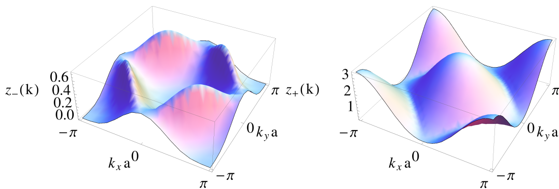
Slika 3.32: Preklopljene spektralne težine z_k za donju i gornju AF vrpcu u korištenom režimu malog procjepa.
