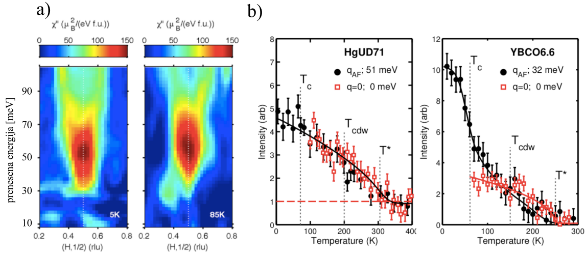
Slika 2.11: Raspršenje neutrons na poddopiranom uzorku Hg1201 kuprata sa T_C = 71 K iz [24]. a) imaginarni dio magnetske susceptibilnosti na 5 K, duboko ispod supravodljivog prijelaza; te 85\text{K} > T_C . Vidljiva je jedna komezurabilna grana iznad komezurabilnog maksimuma oko 50 meV, bez znatnog pojačanja signala na niskim energijama ili pojave nekomezurabilne rezonancije poznate iz drugih kuprata. b) Usporedba temperaturne ovisnosti q = 0 i q = Q_{AF} signala za YBCO i Hg1201: u Hg1201 je Q_{AF} signal izrazito neosjetljiv na supravodljivi prijelaz.
