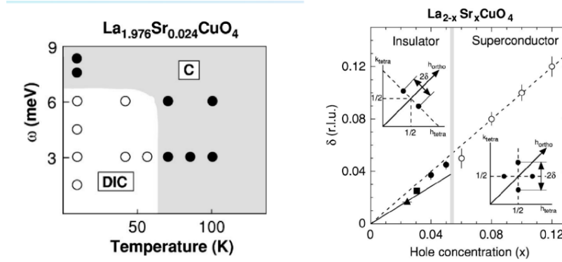
Slika 2.9: Valni vektori magnetskog nekomenzurabilnog uređenja u LSCO-u, preuzeti iz [22]. Lijevo: fazni dijagram pojave dijagonalno nekomenzurabilnog signala u neutronsom rasprešenju za uorak iz-razito niskog dopiranja - na visokim frekvencijama i temperaturama signal je komenzurabilan. Desno: ovisnost iznosa i orijentacije nekomenzurabilnog valnog vektora o dopiranju.
