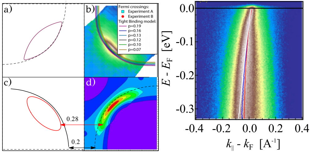
Slika 4.6: Lijevo: ARPES Fermijeva ploha Hg1201 blizu optimalnog dopiranja te nekoliko prikaza prilagodbi korištenih u ovom radu. a) Prilagodba s \mathbf{k} -ovisnim procjepom, većim oko vH točaka, daje premalu zakrivljenost lukova blizu hotspotova ; b) eksperimentalna slika iz [45] s nekoliko prilagodbi za različita dopiranja iz originalnog članka, u kojima nije korišten procjep; c) prilagodba s konstantnim procjepom \Delta_0 = 0.035 eV. d) obojeni prikaz intenziteta na Fermijevoj energiji za prilagodbe bez procjepa, ali s \mathbf{k} -ovisnim gušenjem - širine spektralnih linija su proporcionalne funkciji (\cos(k_x) - \cos(k_y))^n , gdje je n = 4 . Ovaj član simulira procese gušenja koji su pojačani oko vH točaka zbog povećane gustoće stanja i dobro opisuje eksperimentalne rezultate. Desno: nagib eksperimentalne Fermijeve plohe iz [45] te naša prilagodba (bijela linija) na srednji nagib u blizini Fermijevog nivoa.
