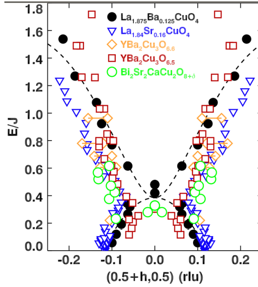
Slika 1.8: Magnetski spektri nekoliko klasa kuprata, skalirani na parametar superizmjene za pripadajuće nedopirane AF spojeve. Točke prikazuju lokalne maksimume intenziteta neutronskeg raspršenja, koji se često poistovjećuju s kolektivnim pobuđenjima (magnonima) s frekvencijom \omega(\mathbf{q}) . Najvažnije opažanje jest pojava tih maksimuma na nekomenzurabilnom valnom vektoru blizu \mathbf{Q}_{AF} te spajanje donjih i gornjih grana magnonske disperzije u komenzurabilnom valnom vektoru na konačnoj frekvenciji \tilde{\omega} .
