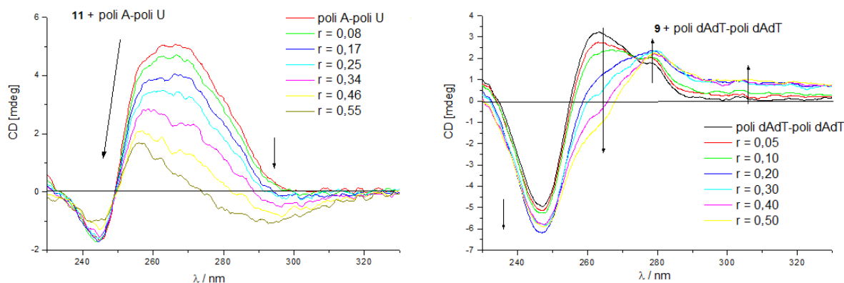
Slika 29. CD titracije: (lijevo) spoja 11 s poli rA-poli rU; (desno) spoja 9 s poli dAdT-poli dAdT. Omjer r=[\text{spoj}]/[\text{polinukleotid}] . LJEVO: Crnim strelicama na grafovima prikazan je: za 250-290 nm pad intenziteta CD spektra karakterističnog za dani polinukleotid bez vezanog liganda; za 290–320 nm negativni ICD male molekule. DESNO: za 250-290 nm pad intenziteta CD spektra karakterističnog za dani polinukleotid bez vezanog liganda; porast CD signala iznad 280 nm posljedica je induciranog CD spektra male molekule (preuzeto iz [99] i prerađeno).
